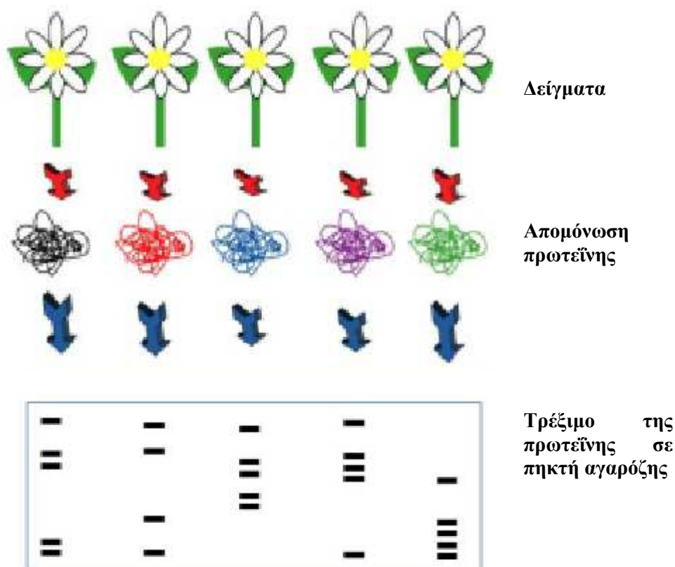
Εικόνα 16: Σύνοψη των γεγονότων που συμβαίνουν σε ένα δείγμα φυτών κατά την ανάλυση ισοενζύμων (Πηγή: www.chembio.uoguelph.ca )
