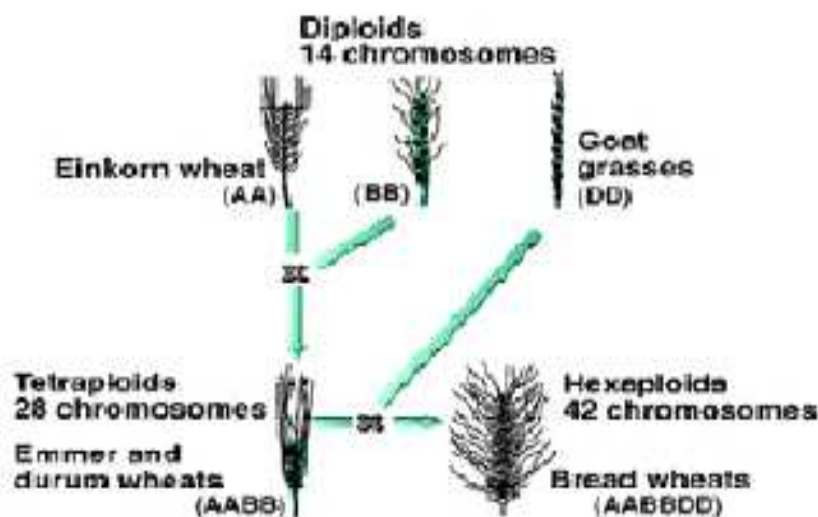
Εικόνα 3: Προέλευση του γονιδιώματος του σιταριού ( Πηγή : eeb.bio.utk.edu.)
