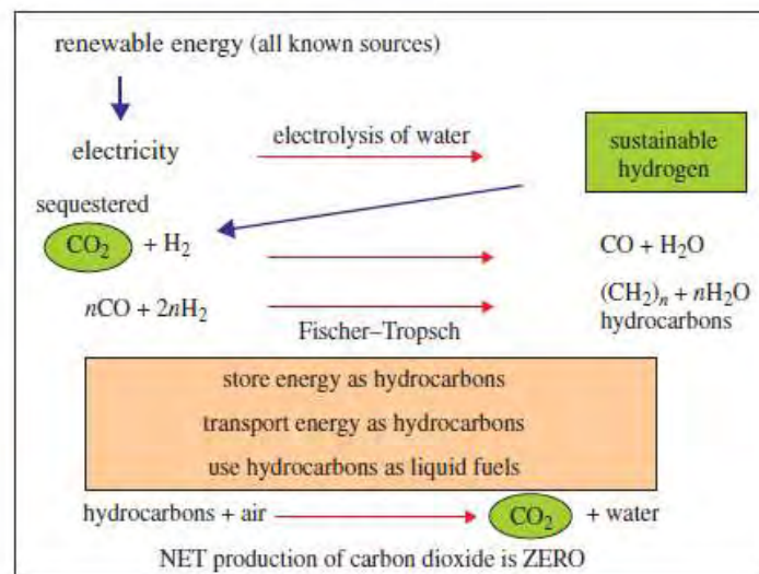
Εικόνα 2.2: Ένας γενικός κύκλος ενέργειας στον οποίο χρησιμοποιείται δεσμευμένο \text{CO}_2 και βιώσιμο ή ανανεώσιμο υδρογόνο για την παραγωγή ανανεώσιμων πηγών ανθρακούχων καυσίμων ή πηγών με ουδέτερο ισοζύγιο άνθρακα. [4]
