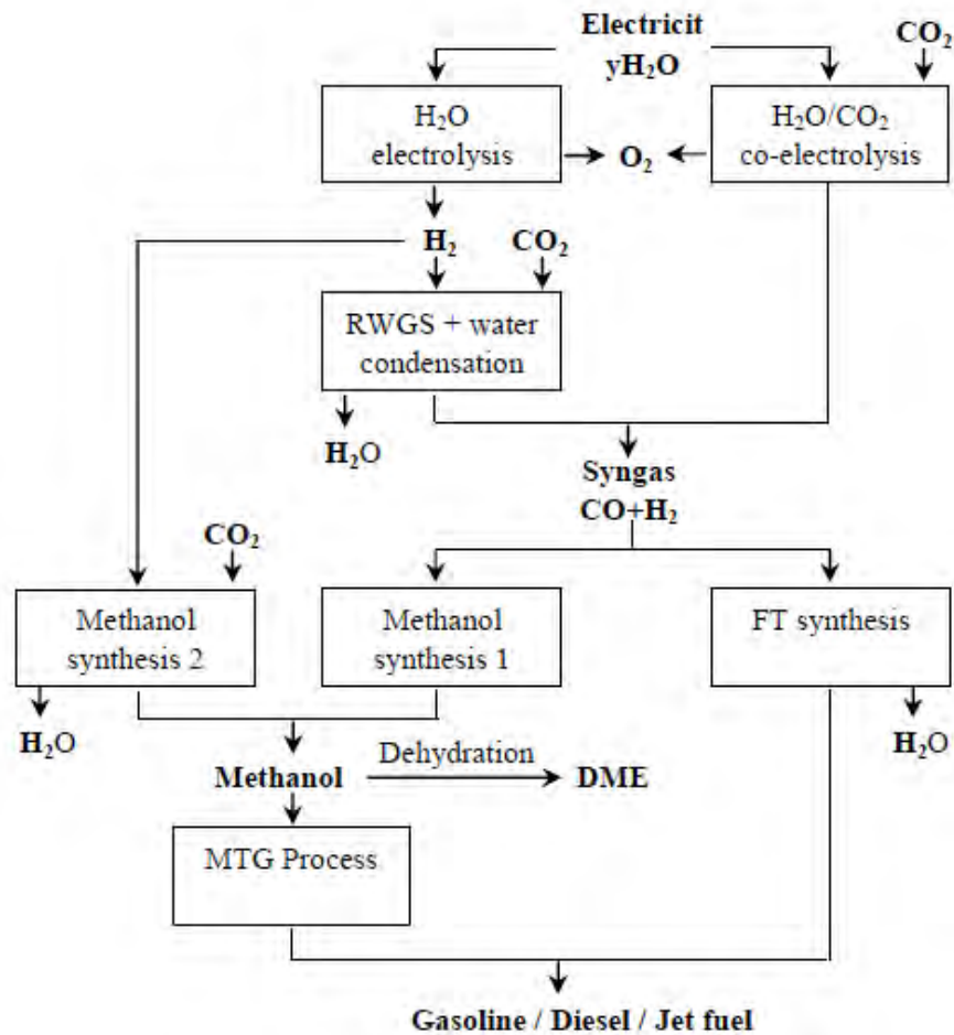
Εικόνα 2.5: Διάφορες διαδρομές για την παραγωγή υγρών καυσίμων από ανανεώσιμες πηγές ηλεκτρικής ενέργειας, \text{H}_2\text{O} και \text{CO}_2 . [6]
