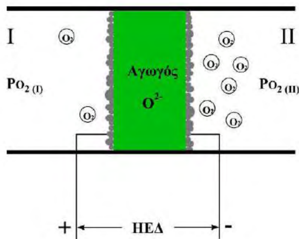
Εικόνα 2.22: Διάταξη Ποτενσιομετρίας Στερεού Ηλεκτρολύτη.
