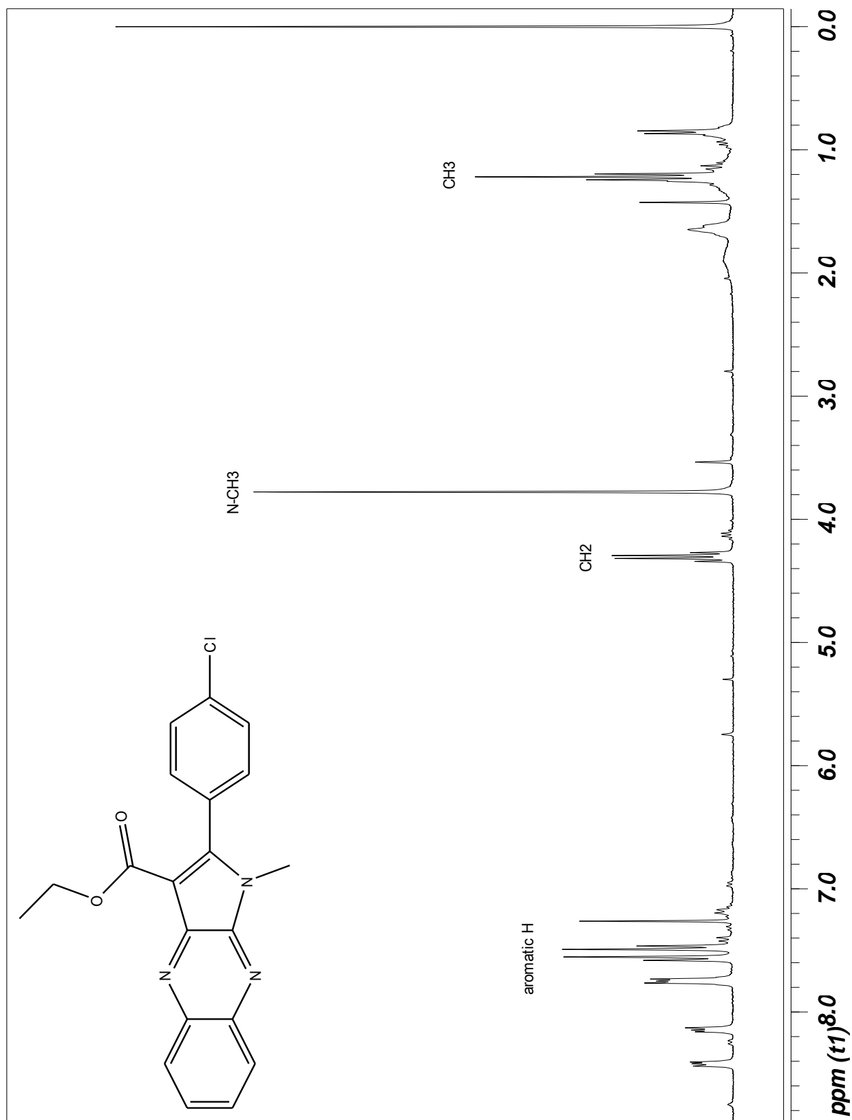
Εικόνα 5.3 Φάσμα ^1\text{H} NMR του αιθυλο-2-(4-χλωροφαινυλο)-1-μεθυλο-1H-πυρρολο[2,3-b]κτινοξαλινο-3-καρβοξυλικού αιθυλεστέρα ( 7 ) σε \text{CDCl}_3 .
