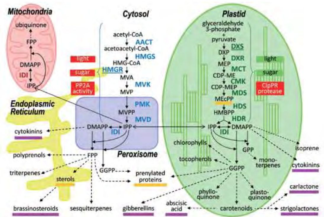
Εικόνα 3: Κυτταρική τοπολογία του μεταβολικού συστήματος των ισοπrenoειδών σε φυτικά κύτταρα όπως συμπεράθηκε από τη διαμερισματοποίηση των ενζύμων του
