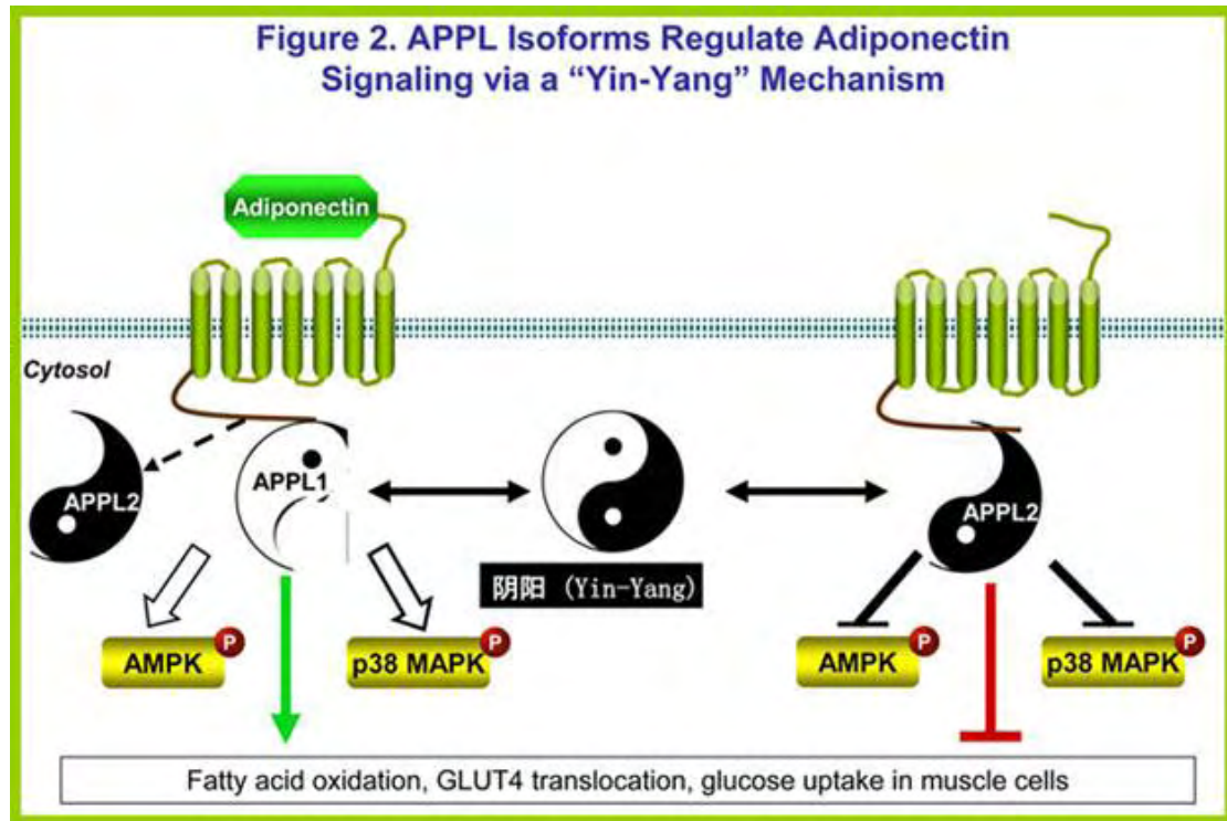
Εικόνα 8: Οι APPL1 / APPL2 ισόμορφες λειτουργούν μεταξύ τους ως ένα ολοκληρωμένο «Yin-Yang» στη σηματοδότηση της αντιπυονεκτίνης.
