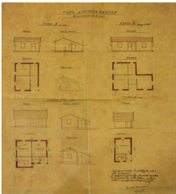
Σχέδιο: τύπος αγροτικού οικισμού, μονοκατοικία (Πηγή: Ιστορικό Αρχείο Προσφυγικού Ελληνισμού)
