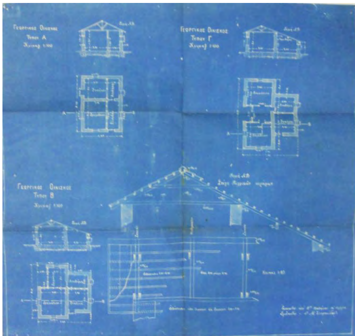
Γεωργικοί οικισμοί τύπου Α,Β,Γ (Πηγή: Ιστορικό Αρχείο Προσφυγικού Ελληνισμού)
