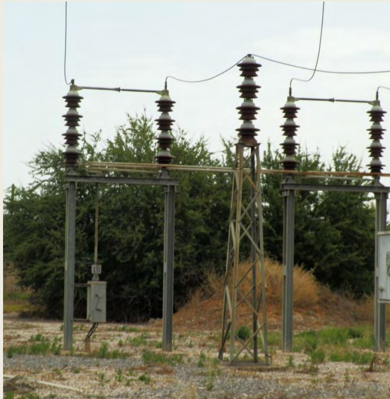
Εικόνα 24: Δίστυλοι αποζεύκτες με περιστρεφόμενες επαφές στον Υ/Σ Οινοφύτων[1]
