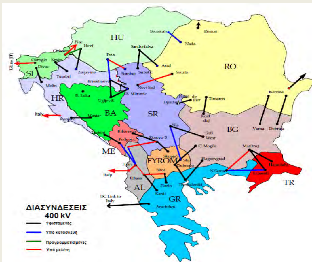
Εικόνα 6: Διασυνδέσεις της Ελλάδος με το εξωτερικό[6]
