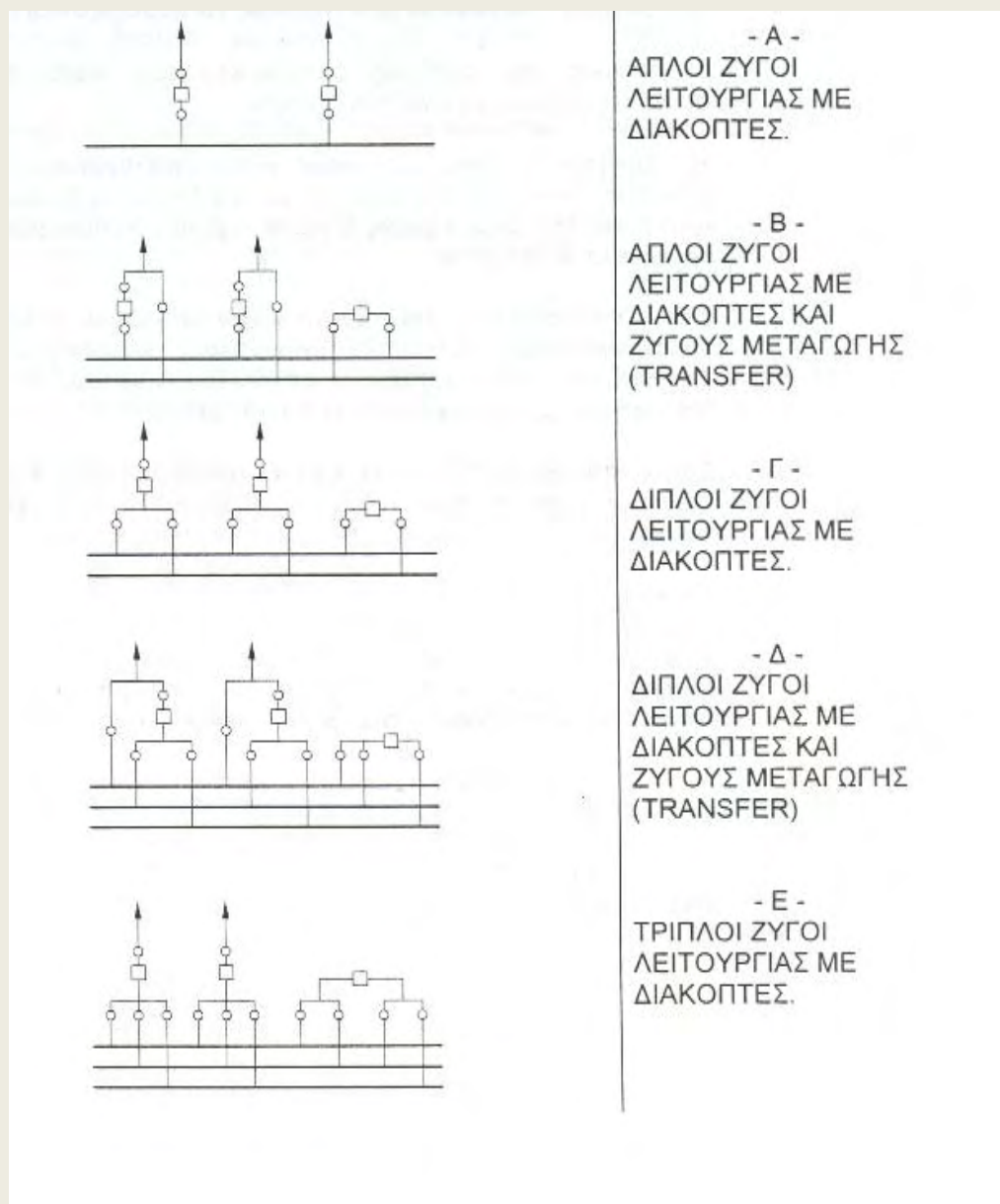
Εικόνα 25:Σχήματα βασικών δομών ζυγών[6]
