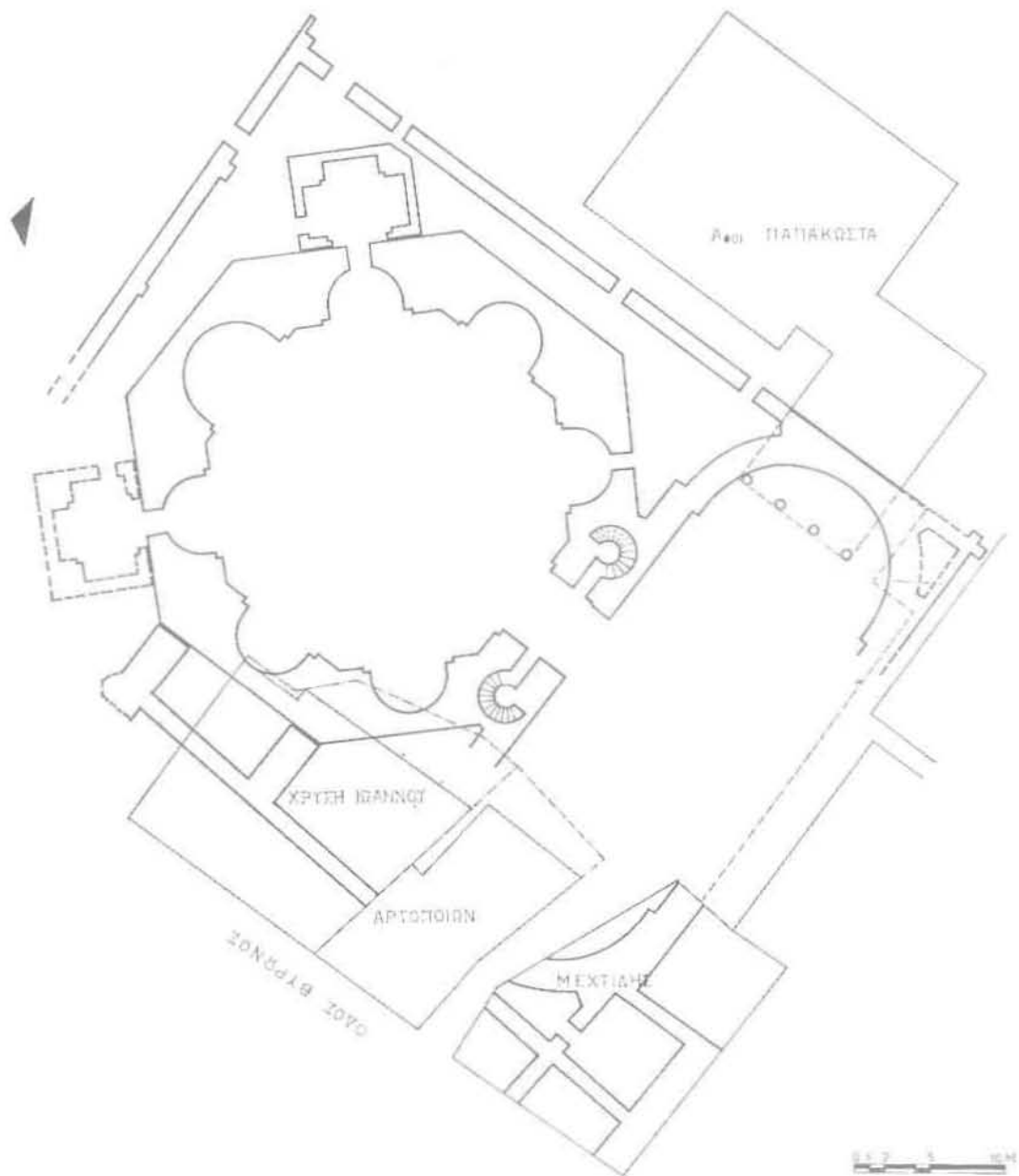
Σχ. 19. Διάταξη της περιοχής του όκταγώνου πριν την έναρξη των ανασκαφών. Κάτωψη.
