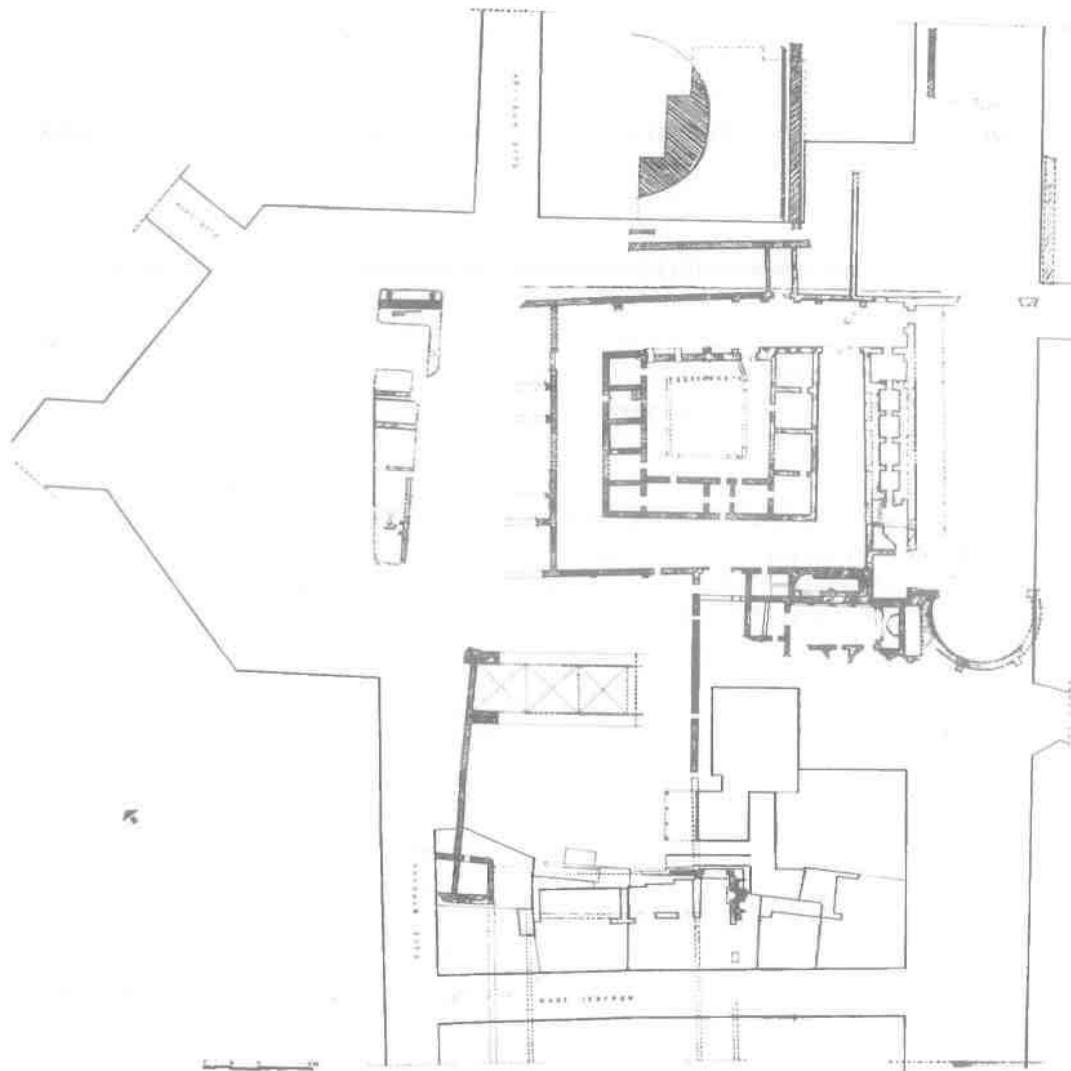
Σχ. 14. Ἀνακτορικό συγκρότημα Γαλερίου στὴν α' φάση (πρὶν ἀπὸ τὴν κατασκευὴ τοῦ ὀκταγώνου). Κάτωψη.
