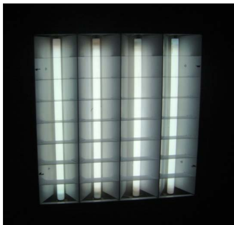
Εικόνα 92: Φωτιστικό σώμα τύπου 1 – Αποτελείται από 4 λαμπτήρες T8 (4*18W)
