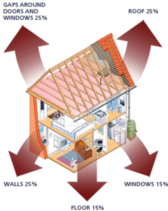
Εικόνα 9. Μέση κατανομή απωλειών ενέργειας από τα διάφορα δομικά στοιχεία ενός κτιρίου.
