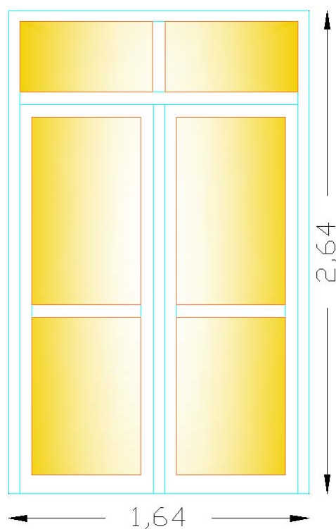
Εικόνα 63: Πόρτα τύπου 10
