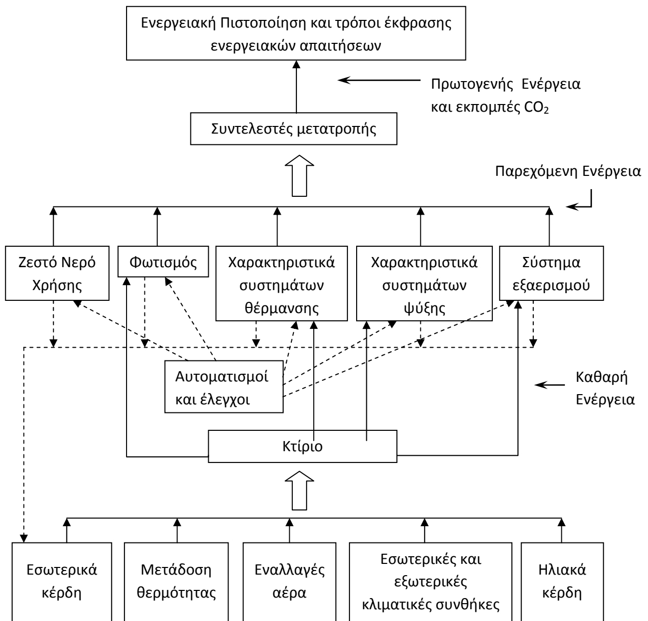
Εικόνα 12: Σύνδεση των ρών της ενέργειας [21]
