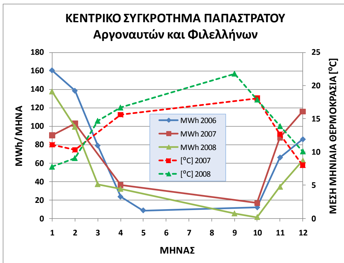
Σχήμα 62: Μηνιαίες καταναλώσεις φυσικού αερίου σε MWh στο Κεντρικό Συγκρότημα Παπαστρατού στην οδό Αργοναυτών και Φιλελλήνων για τα έτη 2006-2008.
