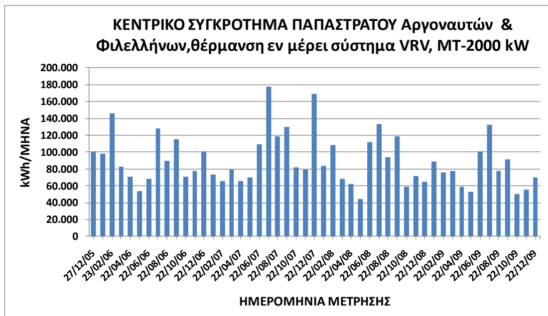
Σχήμα 20: Κεντρικό Συγκρότημα Παπαστρατού Αργοναυτών & Φιλελλήνων MT-2000 kW.
