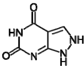
Οξυπουρινόλη
