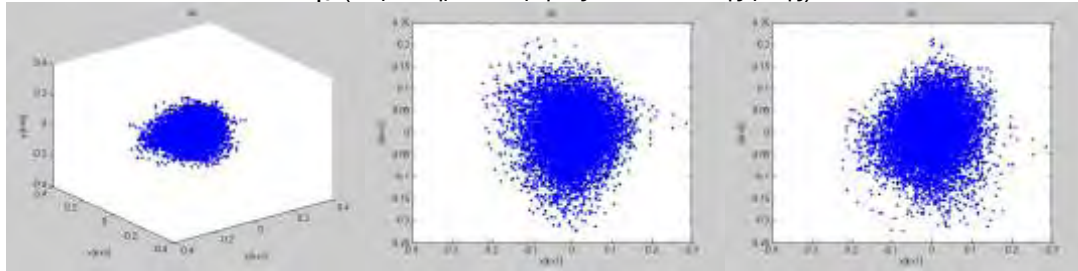
q 7 (Αριθμός Reynolds)
