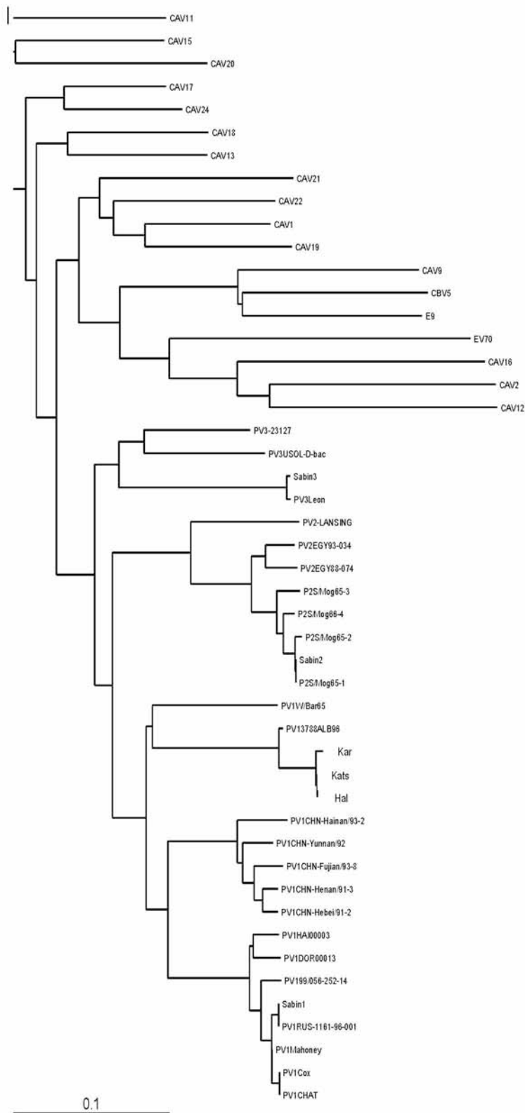
Εικόνα 3.2. Φυλογενετικό δέντρο της VP4 γονωμικής περιοχής για τα στελέχη Kats , Hal και Kar .
