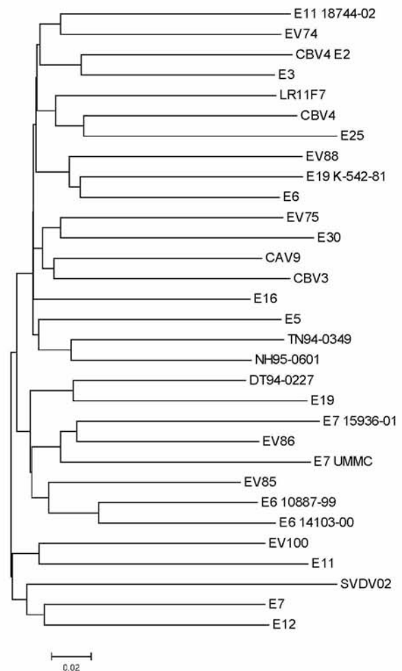
Εικόνα 3.18. Φυλογενετικό δέντρο της 2Α περιοχής για το στέλεχος LR11F7.
