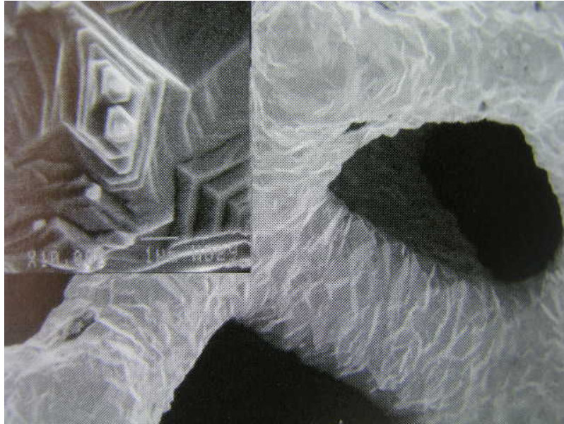
ΕΙΚΟΝΑ 53. Μικροφωτογραφία της επιφάνειας του TMT όπου διακρίνεται η διαμορφωση κρυσταλικής στοιβάδας Τανταλίτη μετά από επεξεργασία με NaOH.
