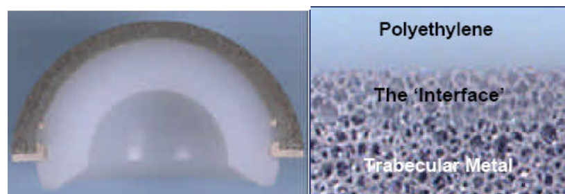
ΕΙΚΟΝΑ 60. Τομή του κυπέλλου και σχηματική αναπαράσταση της διεπιφάνειας TMT-πολυαιθυλενίου. Το πλαστικό διεισδύει στους πόρους και σταθεροποιείται με πίεση.
