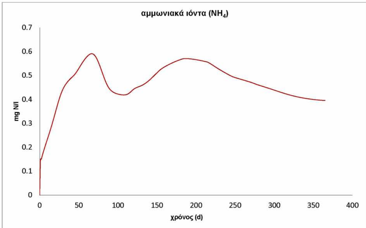
Διάγραμμα 4.19: αμμωνιακά ιόντα (NH 4 )- χρόνος, για ένα έτος προσομοίωσης
