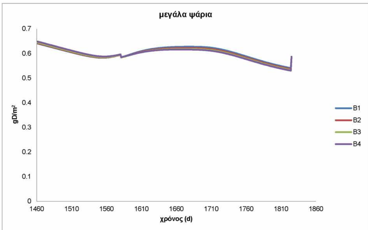
Διάγραμμα 9.18 : μεγάλα ψάρια- χρόνος για ένα έτος προσομοίωσης για τα σχέδια διαχείρισης Β
