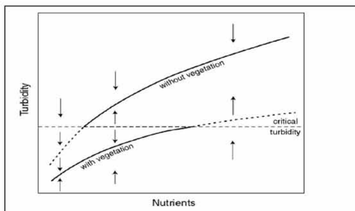
Εικόνα 2.13: Γραφική παράσταση της «θεωρίας των εναλλακτικών σταθερών καταστάσεων» όπου φαίνεται η σχέση μεταξύ της θολότητας και της συγκέντρωσης των θρεπτικών αλάτων σε δύο διαφορετικές καταστάσεις, με ή χωρίς υδρόβια βλάστηση. Οι καμπύλες δείχνουν μεταξύ θρεπτικών και θολότητας σε λίμνες όπου κυριαρχεί το φυτοπλαγκτόν (πάνω καμπύλη) ή τα υδρόβια μακρόφυτα (κάτω καμπύλη). (Scheffer et al., 1993)
