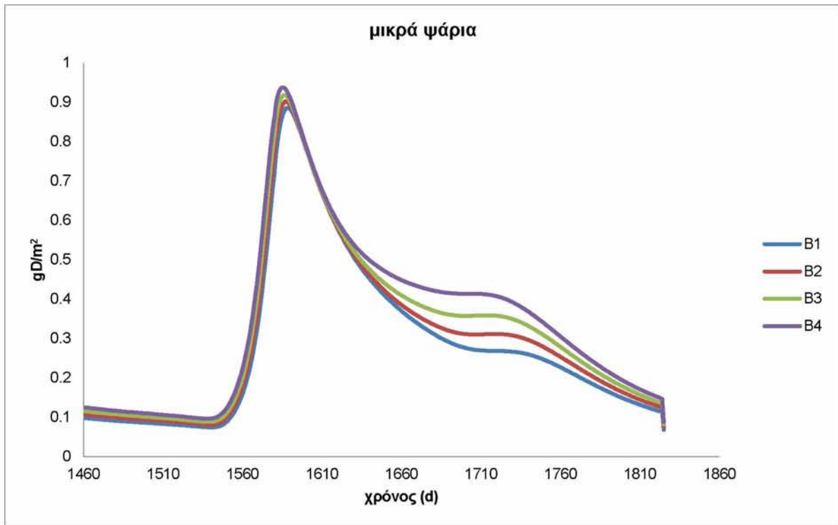
Διάγραμμα 9.1117 : μικρά ψάρια- χρόνος για ένα έτος προσομοίωσης για τα σχέδια διαχείρισης Β
