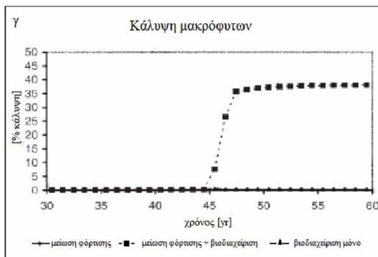
Διαγράμματα 3.7: Προσομοιώσεις διάφορων επιλογών διαχείρισης για τη μέση λίμνη, βάθους 2 m. Η λίμνη αρχικά μετατράπηκε από διαγνή σε θολερή μέσω αύξησης της φόρτισης σε θρεπτικά και ακολούθησαν 3 επιλογές: (1) μείωση της φόρτισης στο αρχικό μέσο επίπεδο, (2) ομοίως συνδυασμένο με βιοδιαχείριση 5 έτη αργότερα και (3) μόνο βιοδιαχείριση συνεχίζοντας την υψηλή φόρτιση. β) χλωροφύλλη-α και γ) κάλυψη μακρόφυτων. (Janse JH, 2005. Model studies on the eutrophication of shallow lakes and ditches. PhD thesis. Wageningen University)
