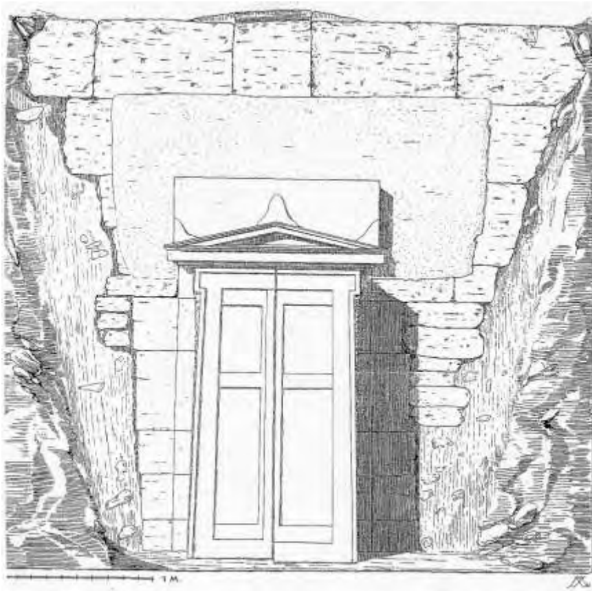
Εικ. 6. Πρόσοψη Μακεδονικού τάφου Αρ. 4
