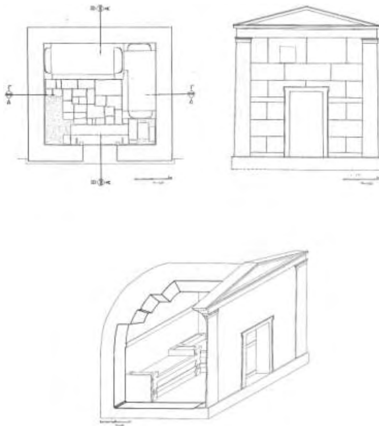
Εικ. 114. Κάτοψη, πρόσοψη και αξονομετρική απόδοση Μακεδονικού τάφου Αρ. 66 (Ποτίδαιας ΙΙ)
