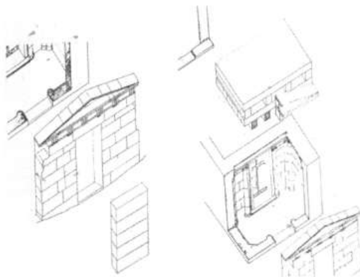
Εικ. 65. Πρόσοψη και προθάλαμος Μακεδονικού τάφου Αρ. 33
