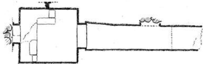
Εικ. 128. Κάτοψη Μακεδονικού τάφου Αρ. 74 (Αμφίπολη ΙΙ)
