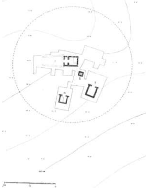
Εικ. 51. Κάτοψη Μακεδονικών τάφων Αρ. 24, 25, 26 τύμβου Μπέλλα
