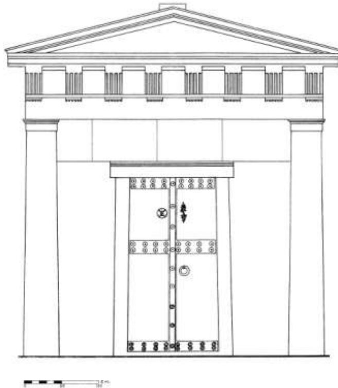
Εικ. 107. Πρόσψη Μακεδονικού τάφου Αρ. 61 (Αγ. Παρασκευή)
