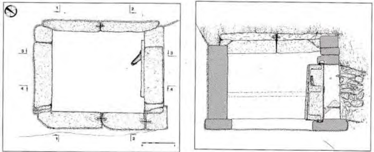
Εικ.4. Κάτοψη και τομή 3-3 Μακεδονικού τάφου Αρ. 2
