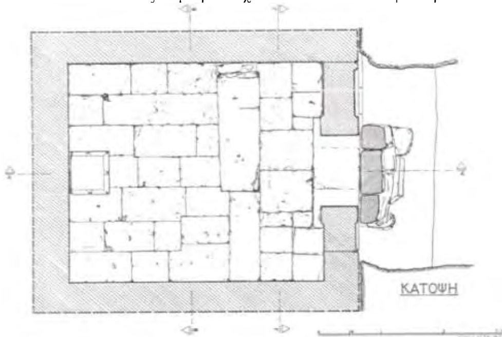
Εικ. 58. Κάτωψη Μακεδονικού τάφου Αρ. 29
