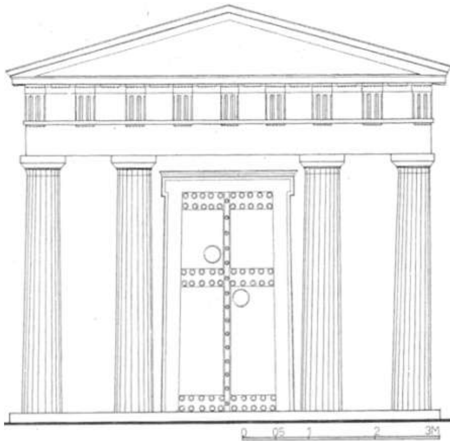
Εικ. 54. Πρόσοψη-αποκατάσταση Μακεδονικού τάφου Αρ. 27
