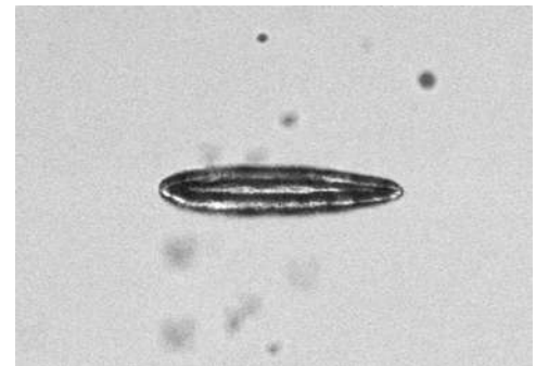
Σχήμα 4.7 Αρχικό σχήμα Φυσαλίδας για παλμού Ενέργειας 100 μJ
