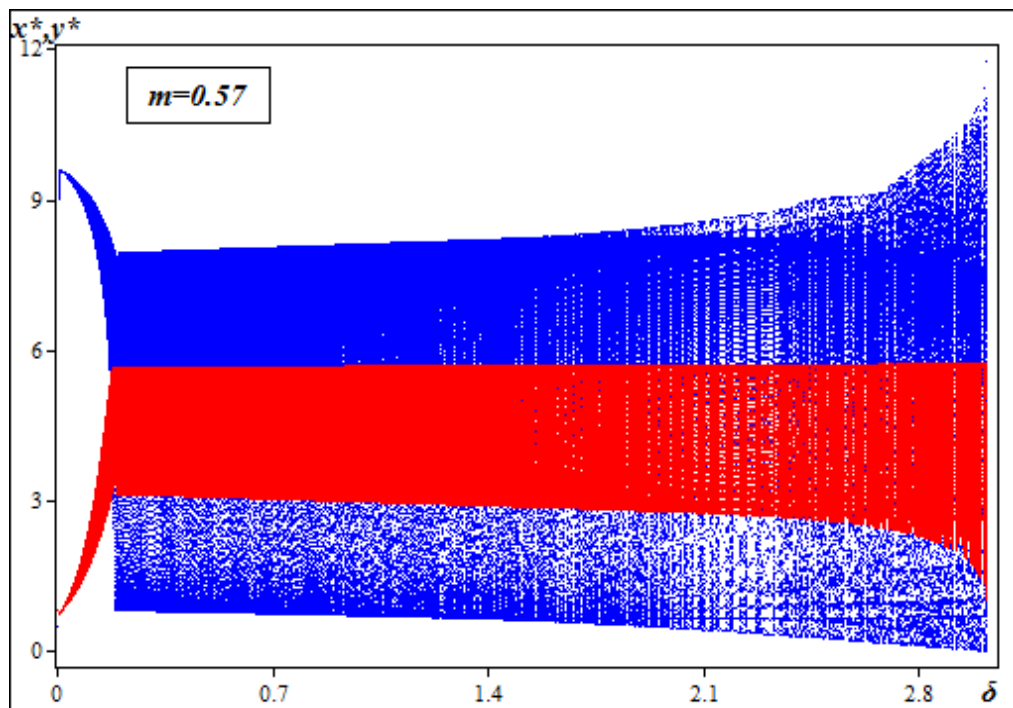
Σχήμα 8.2 Διάγραμμα διακλάδωσης θηρευτή-θηράματος για 0 < \delta < 3,05
