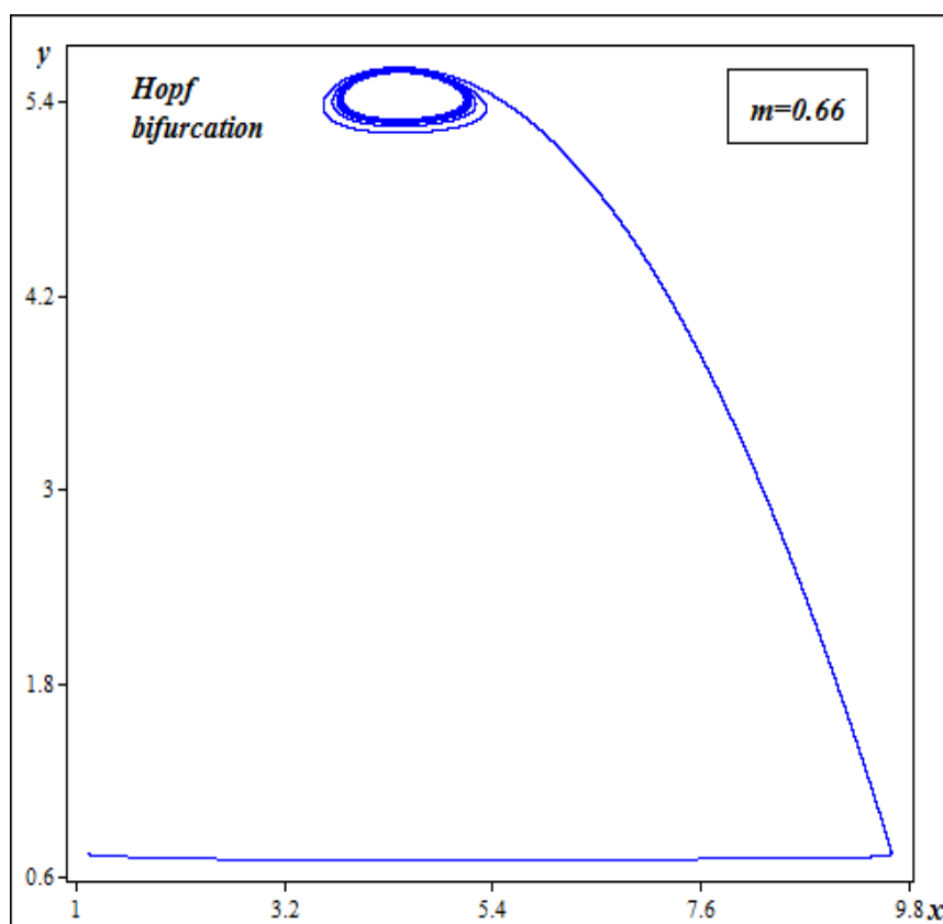
Σχήμα 7.3. Διάγραμμα φάσεων για m = 0,66
