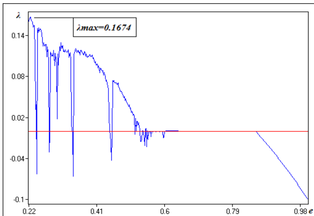
Σχήμα 5.5 Διάγραμμα εκθέτη Lyapunov με \varepsilon ( 1 \rightarrow 0,22 ).
