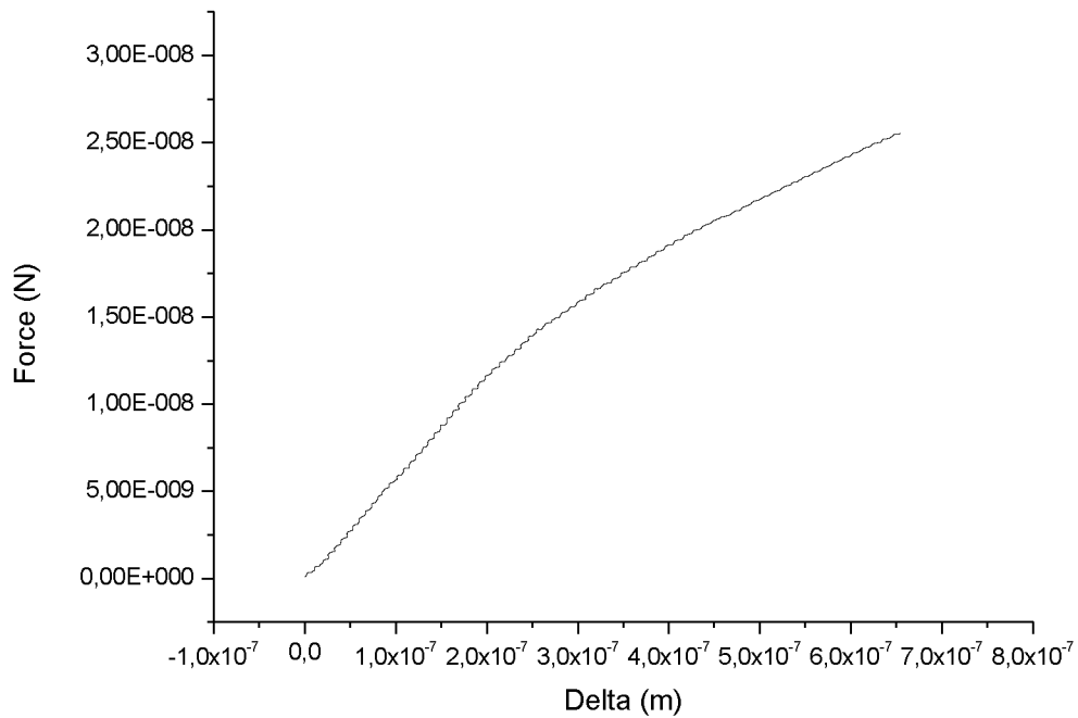
Σχήμα 50: Διάγραμμα δύναμης-μετατόπισης
