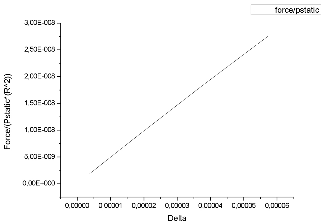
Σχήμα 17:Γραμμική περιοχή
