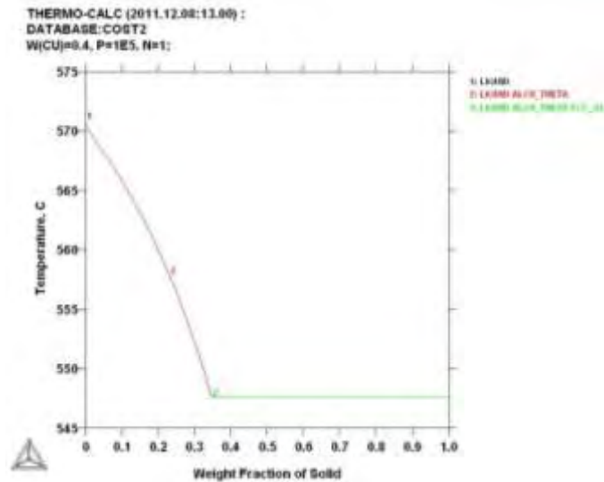
Σχ. 27: Πορεία στερεοποίησης για σύσταση 40%Cu
