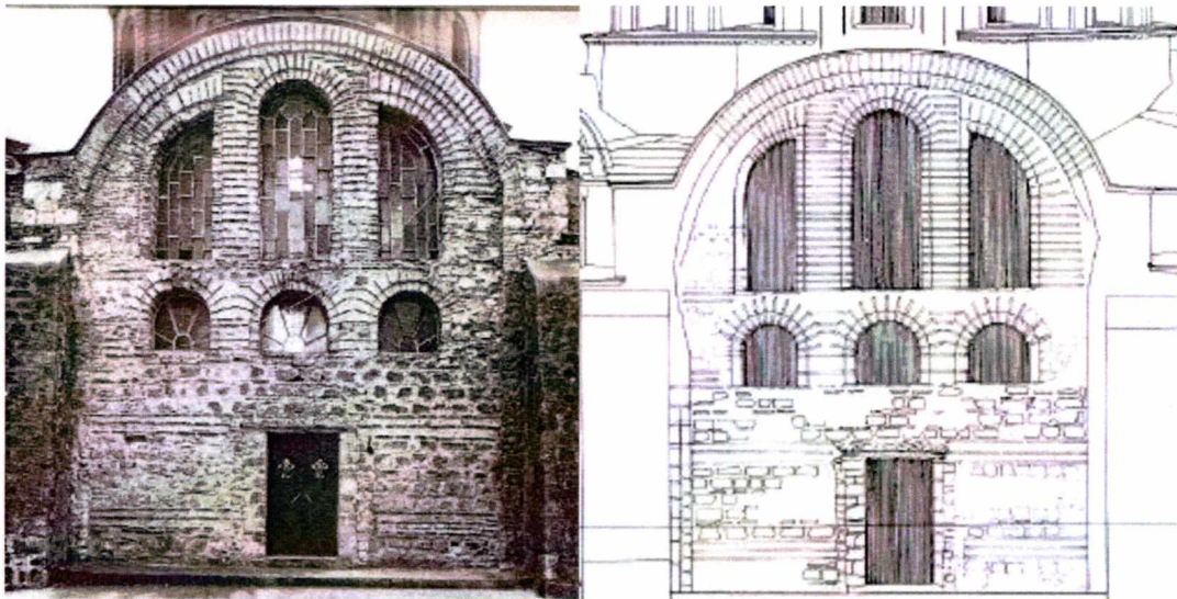
Εικόνα 44 : Λεπτομέρεια βόρειας όψης καθολικού (αριστερά) και λεπτομέρεια σχεδιαστικής απόδοσης βόρειας όψης καθολικού (δεξιά). Πηγή εικόνων: Sinos 1985
