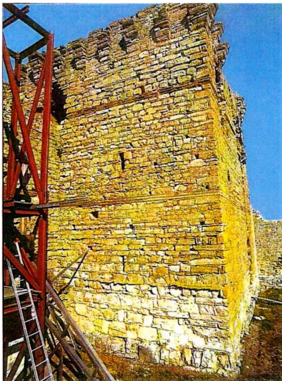
Εικόνα 30: Πύθιο. Μεγάλος πύργος, Νότια πλευρά (αριστερά). Σχεδιαστική απόδοση παραθύρων νότιας πλευράς. όψη από το εσωτερικό και το εξωτερικό (δεξιά). Πηγή εικόνας: Τσουρής, Μπρίκας 2002
