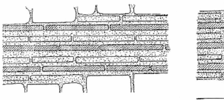
Εικόνα 25: Σχεδιαστική απόδοση της τοιχοποιίας του φρουρίου του Πυθίου. Πηγή εικόνας: Τσουρής, Μπρίκας 2002
