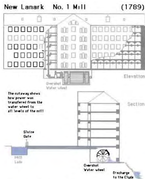
Εικόνα 6: Τρόπος λειτουργίας του μύλου
