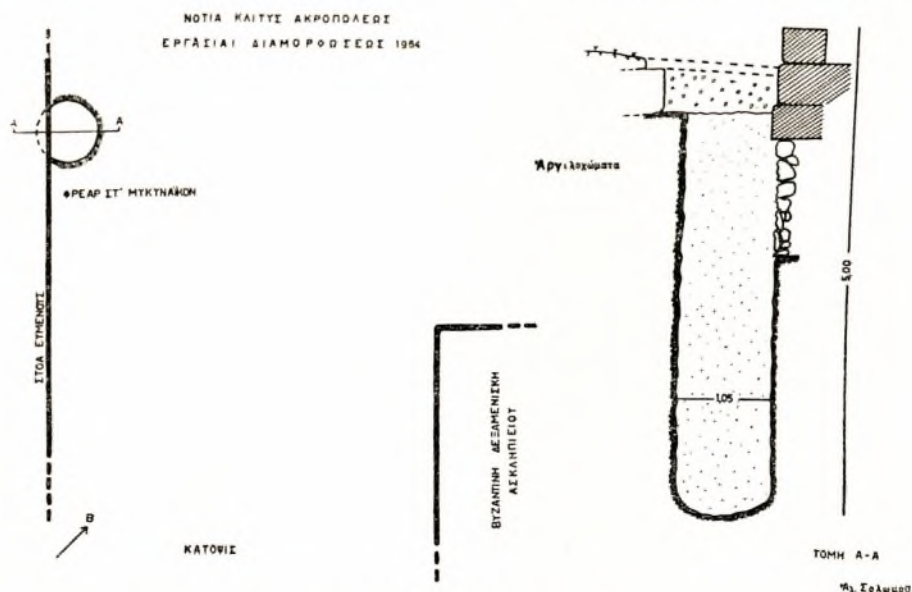
Σχέδ. 5. Κάτωπις καὶ τομὴ τοῦ Β. τῆς Στοᾶς Εὐμένουσ μυκηναϊκοῦ φρέατος ΣΤ'
