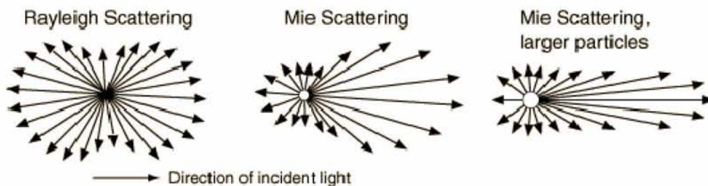
Σχήμα 2.9 : Σκέδαση Rayleigh και Mie (hyperphysics.phy)
