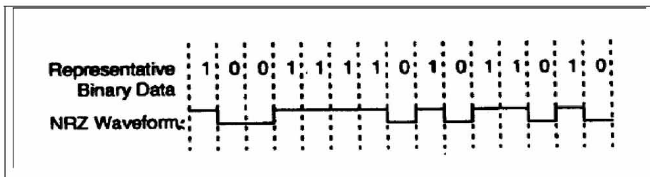
Σχήμα 3.2 : Κυματομορφή NRZ (Lambert & Casey, 1995)
