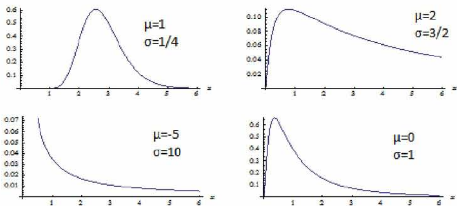
Σχήμα 4.1 : Γραφικές παραστάσεις της συνάρτησης πυκνότητας πιθανότητας
