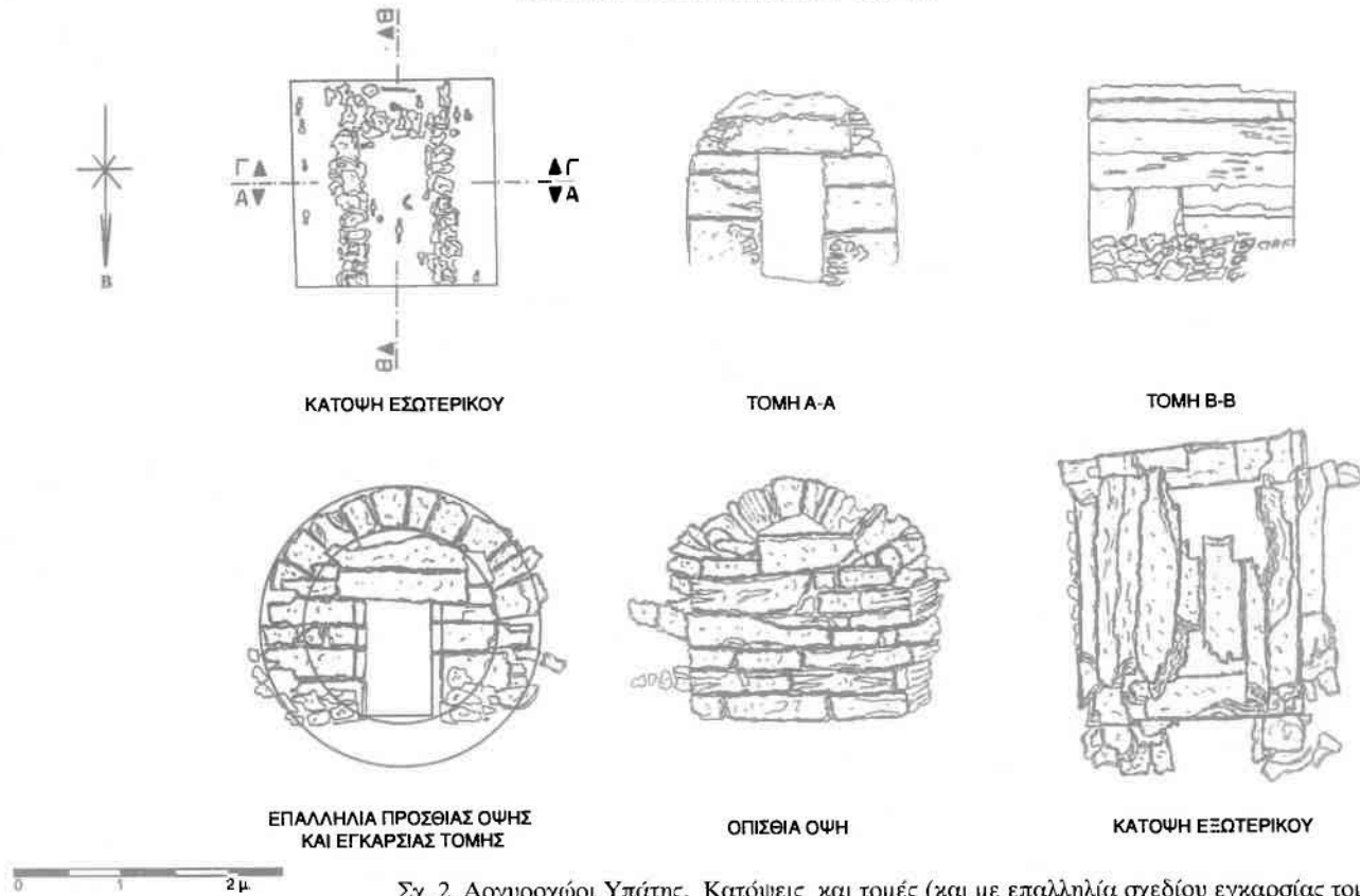
Σχ. 2. Αργυροχώρι Υπάτης. Κατόψεις και τομές (και με επαλληλία σχεδίου εγκάρσιας τομής και πρόσοψης) του κτιστού, καμαροσκεπούς τάφου.
