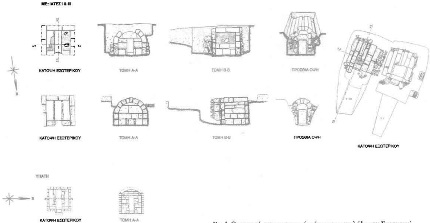
Σχ. 4. Οι κτιστοί, καμαροσκεπείς τάφοι στην κοιλάδα του Σπερχείου με κλίνες εκατέρωθεν του διαδρόμου του θαλάμου.
