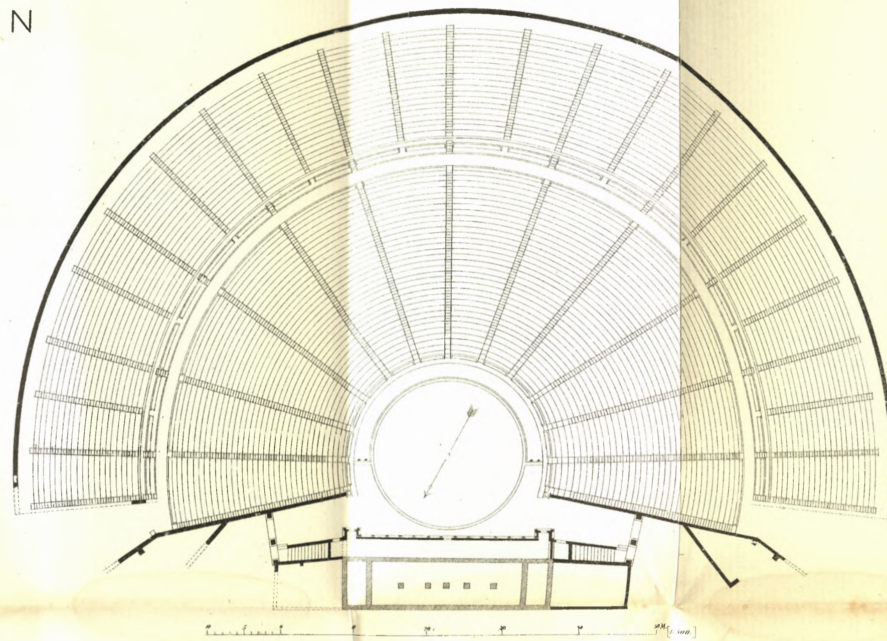
1. Κάτοψη του θεάτρου.
