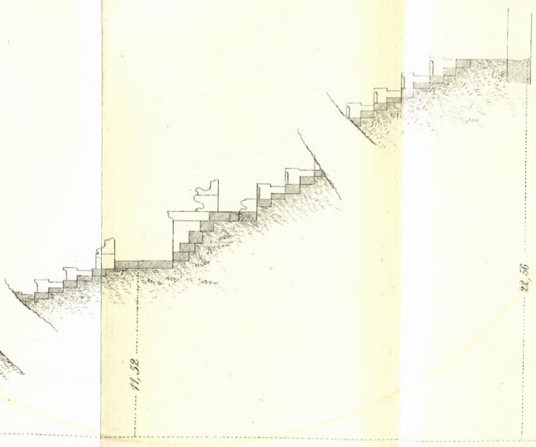
2. Τομή του τοίχου [1:100]
