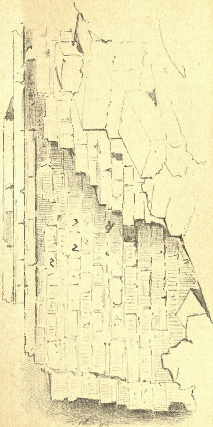
Ἀποψη μέρους τῆς βορείας πλευρᾶς τοῦ Γεφενάτου τοῦ ἐν Ἐλευσίῃ Ναοῦ.
