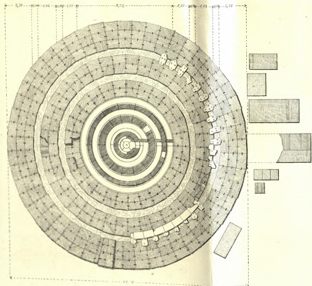
1 Ἐπίγειος τοῦ οἰκοδομήματος
