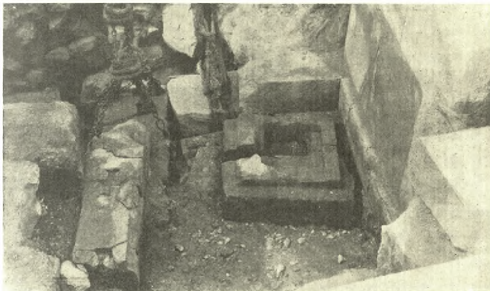
Εἰκ. 13. Ἡ πρὸς δυσμὰς καὶ μεσημβρίαν εὐθυνηρία τοῦ κτίσματος. Ἀποψις τοῦ ἀποκαλυφθέντος βόθρου.
