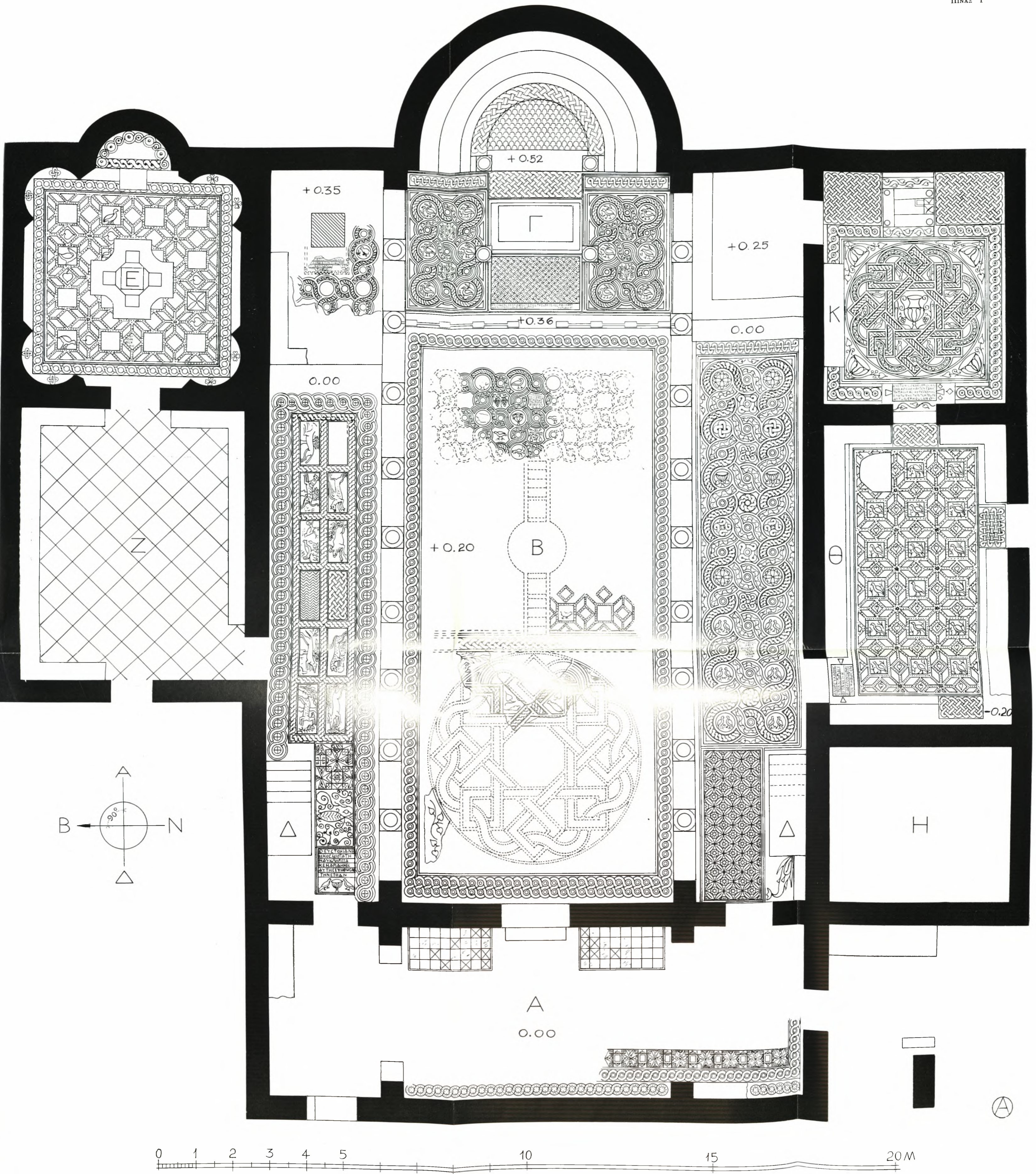
Κάτωψις της βασιλικής του Μαστιγάρη μετά της διακοσμήσεως τών δαπέδων αυτής.
