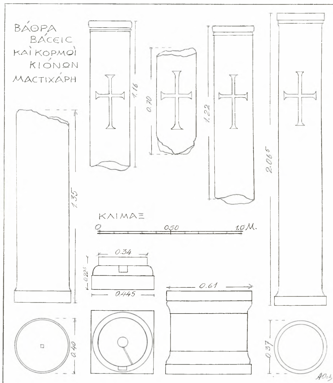
Εἰκ. 10. Βάθρον, βάση καὶ κορμοὶ κίωνων τῆς βασιλικῆς τοῦ Μαστιχάρη.
