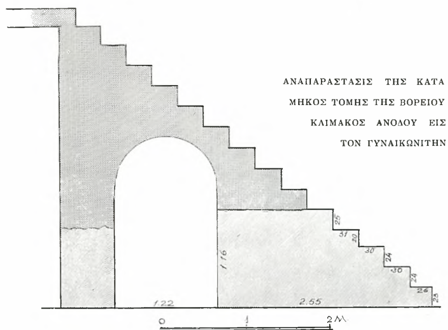
Εἰκ. 20. Τομή κατὰ μῆκος τῆς βορείου κλίμακος ἀνόδου εἰς τὸν γυναικωνίτην. Τὰ σωζόμενα μέρη δηλοῦνται διὰ διαγραμμίσσεως.
