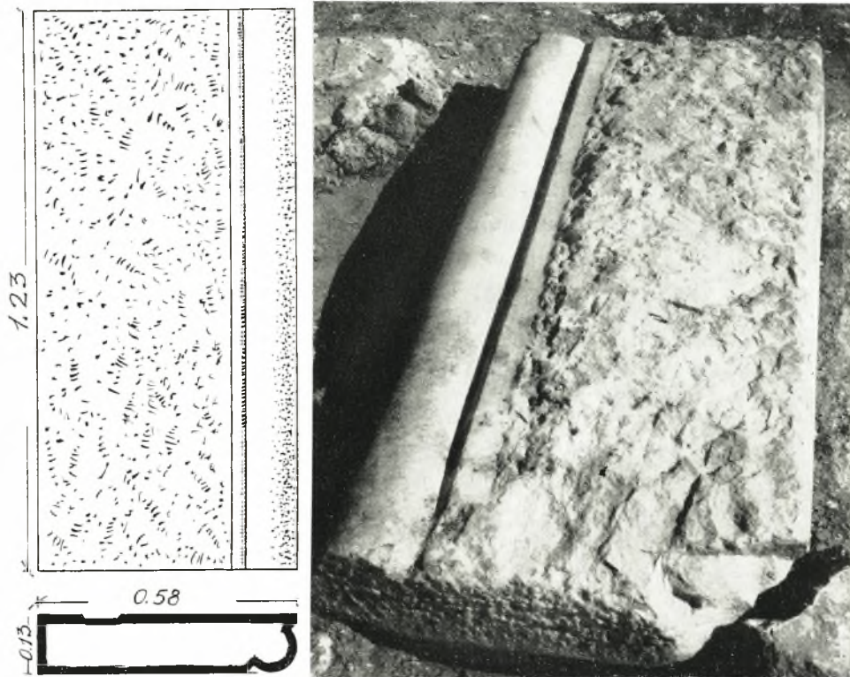
Εἰκ. 17. Κάτοψις, τομὴ καὶ προοπτικὴ ὄψις τοῦ κοσμητοῦ.
