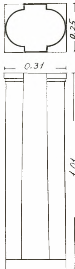
Εἰκ. 15. Ὁριζοντία τομὴ καὶ πλάγια ὄψις διαχωριστικοῦ κιονίσκου παραθύρου.
