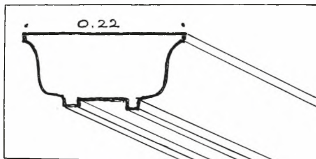
Εἰκ. 31. Μαρμαρινὴ στέψις θωρακίου.
