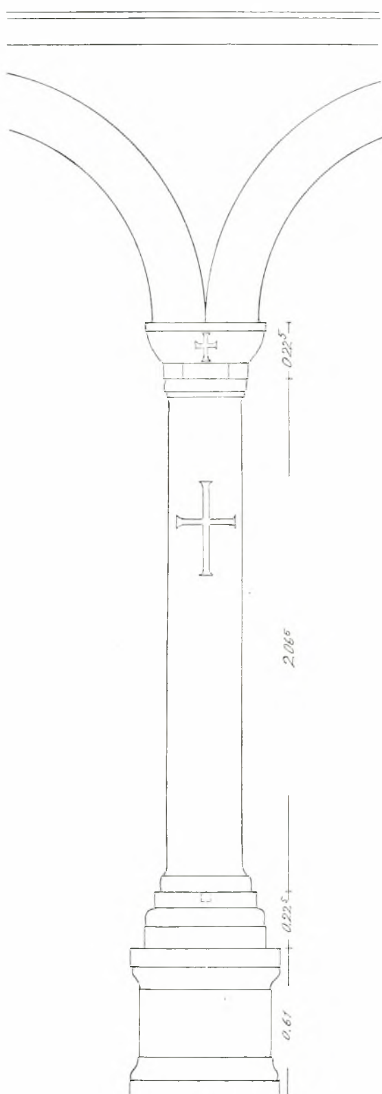
Εἰκ. 14. Ἀναπαράστασις ἑνὸς τῶν στηριγμάτων τῶν κινοστοιχιῶν μετὰ τῶν ἐπ' αὐτοῦ τόξων.
