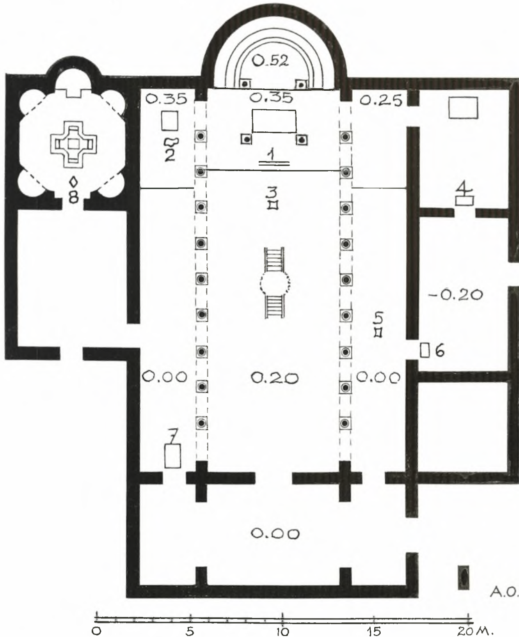
Εἰκ. 89. Κάτωψις τῆς βασιλικῆς ἐμφαίνουσα τὴν θέσιν τῶν ψηφιδωτῶν ἐπιγραφῶν διὰ τῶν ἀριθμῶν 1 ἕως 8. τῶ ναῶ, σημειοῦνται ἐπὶ τῆς παρατιθεμένης κατόψεως αὐτοῦ (εἰκ. 89) διὰ τῶν ἀριθμῶν 1 ἕως 8. Ἐπὶ τοῦ αὐτοῦ σχεδίου σημειοῦνται καὶ τὰ ὑψόμετρα τῶν διαφόρων χώρων.
