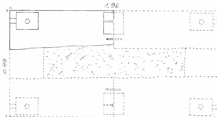
Εἰκ. 25. Ἀναπαράστασις τῆς βάσεως τῆς Ἁγ. Τραπέζης.
