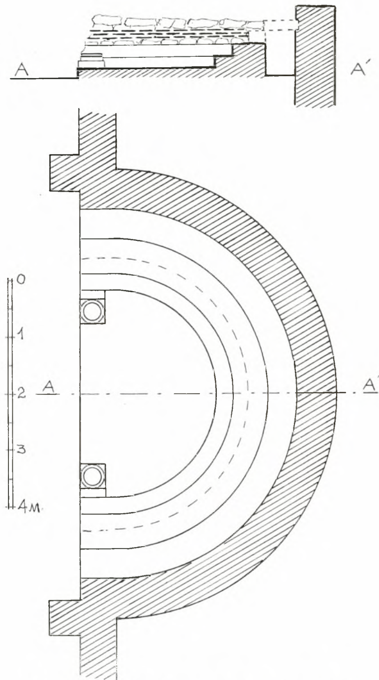
Εἰκ. 22. Κάτοψις καὶ τομὴ κατὰ μῆκος τῆς ἀψίδος τοῦ ἱεροῦ.
