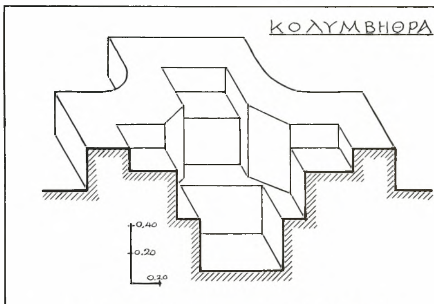
Εἰκ. 43. Ἴσομετρικὴ ἀναπαράστασις καὶ τομὴ τῆς κολυμβήθρας.
