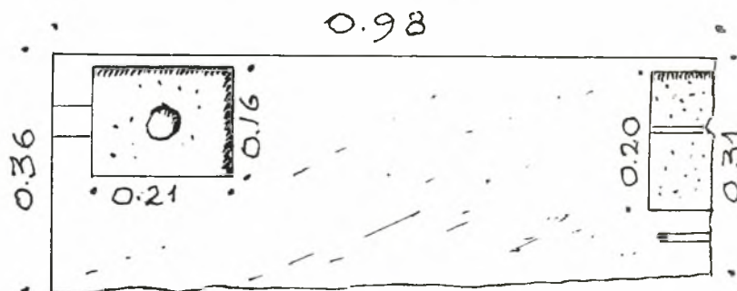
Εἰκ. 24. Τεμάχιον ἐκ τῆς μαρμαρίνης βάσεως τῆς Ἁγ. Τραπέζης.
