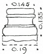
Εἰκ. 26. Βᾶσις κιονίσκου τῆς Ἀγ. Τραπέζης.
