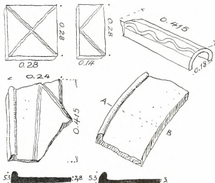
Εἰκ. 35. Πλίνθοι τῆς τοιχοδομίας (ἄνω ἀριστερᾶ) καὶ κέραμοι τῆς στέγης καὶ τοῦ τεταρτοσφαιρίου.
