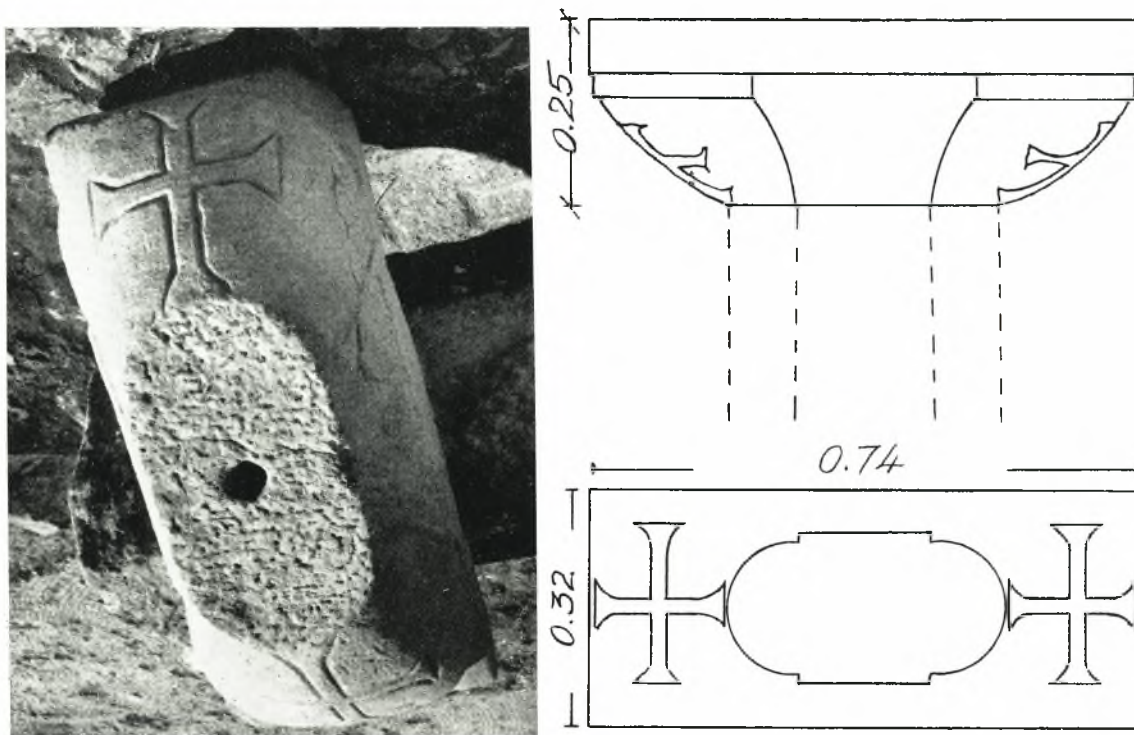
Εἰκ. 23. Κιονόκρανον ἐκ τοῦ παραθύρου τοῦ ἱεροῦ.
