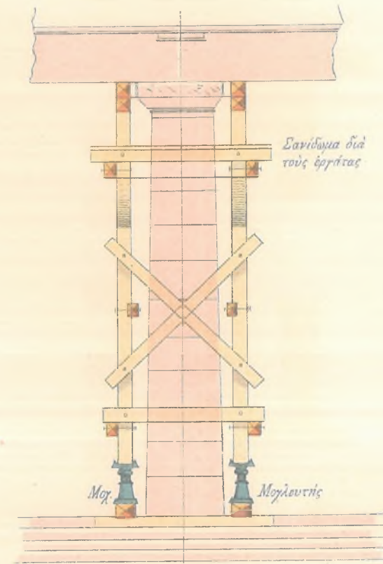
ΙΚΡΙΑ ΠΡΟΣ ΕΠΙΣΚΕΥΗΝ ΤΩΝ ΕΠΙΚΡΑΝΩΝ ΤΩΝ ΚΙΟΝΩΝ
