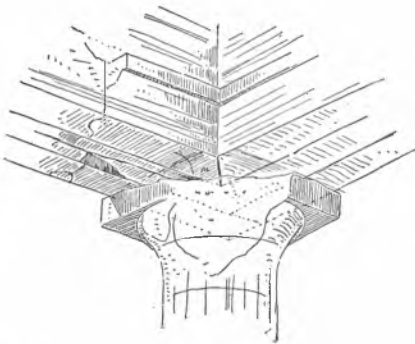
Σχῆμα 10. Βορειοδυτικὸς γωνιαῖος κίον τοῦ ὀπισθοδόμου. Ἐποψὶς ἐκ τῶν ἐνδόν.
