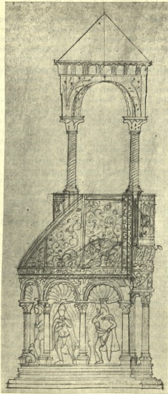
Εικ. 4. Ἀποκατάσταση τοῦ Ἀμβωνοῦ τῆς Θεσ/νίκης. Πλαγία ὄψις.
