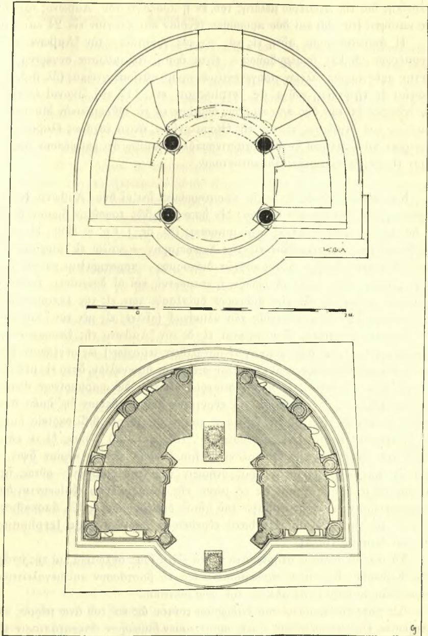
Εἰκ. 1-2. Κάτοπις βάσεως καὶ ἄνω δαπέδου τοῦ Ἄμβωνος τῆς Θεσσαλονίκης.
