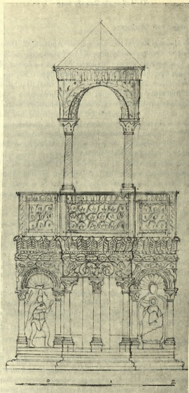
Είκ. 3. Ἀποκατάσταση τοῦ Ἄμβωνος τῆς Θεσσαλονίκης. Κυρία ὄψις.
