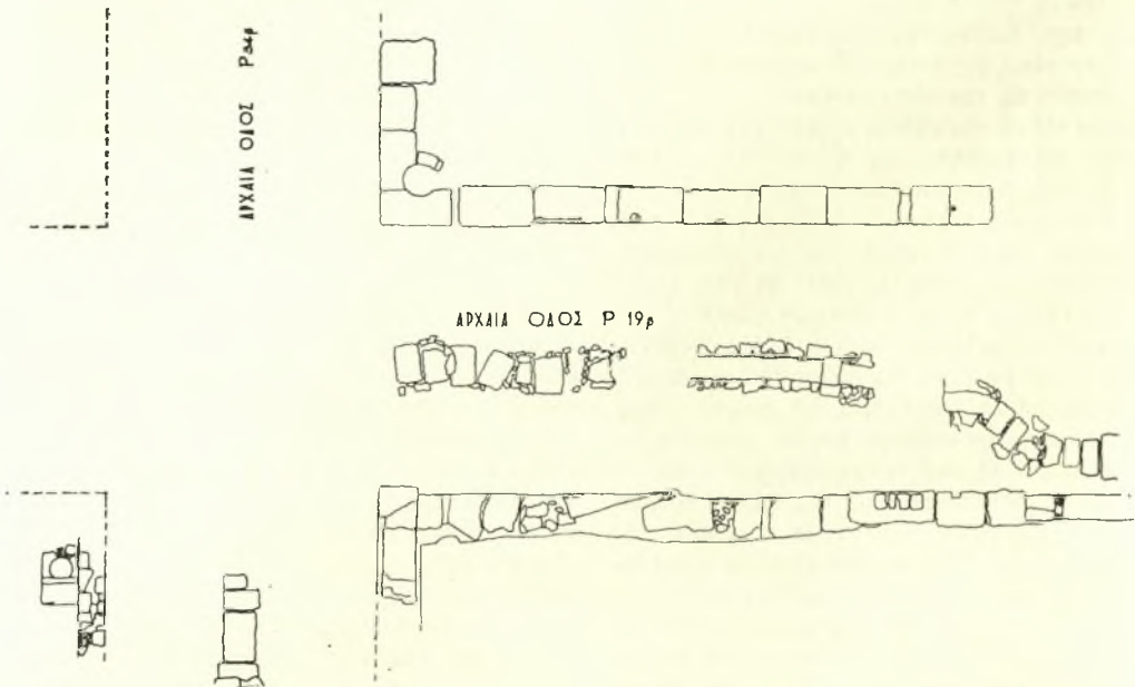
Σχέδ. 6. Ἀνασκαφὴ οἰκοπέδου Ἀναστασιάδη. Διασταύρωσις ἀρχαίων ὁδῶν P19β και P34β
