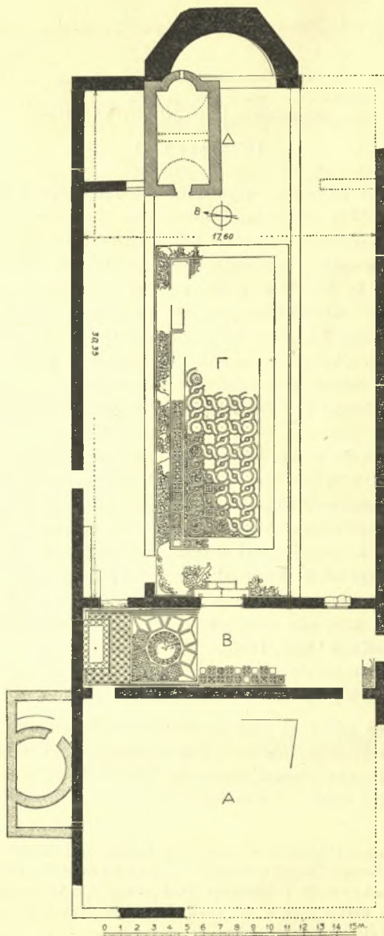
Εἰκ. 1. Κάτοψις τῆς βασιλικῆς Α τῆς Χερσονήσου ἄνευ τοῦ ΝΑ. προσκτίσματος (Α αἶθριον, Β νάρθηξ, Γ κυρίως ναός, Δ πρεσβυτήριον).
