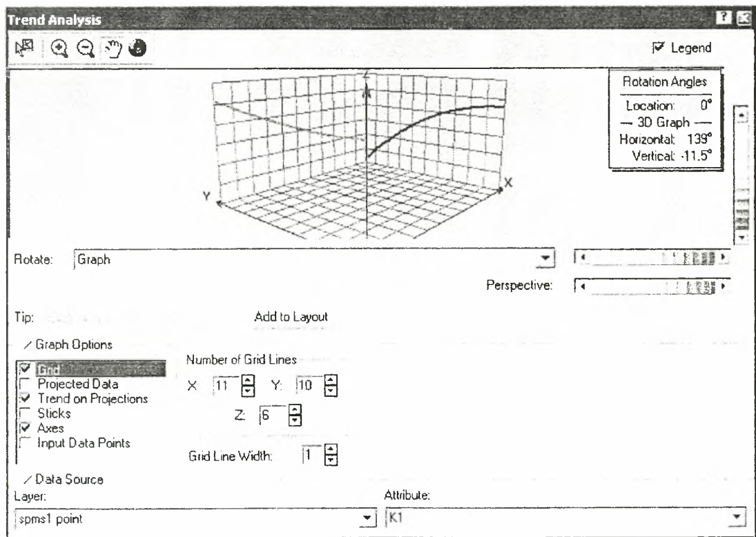
Ανάλυση της τάσεως των τιμών του καλίου στα φύλλα αμπέλου (1 η Δειγματοληψία) στην περιοχή μελέτης
