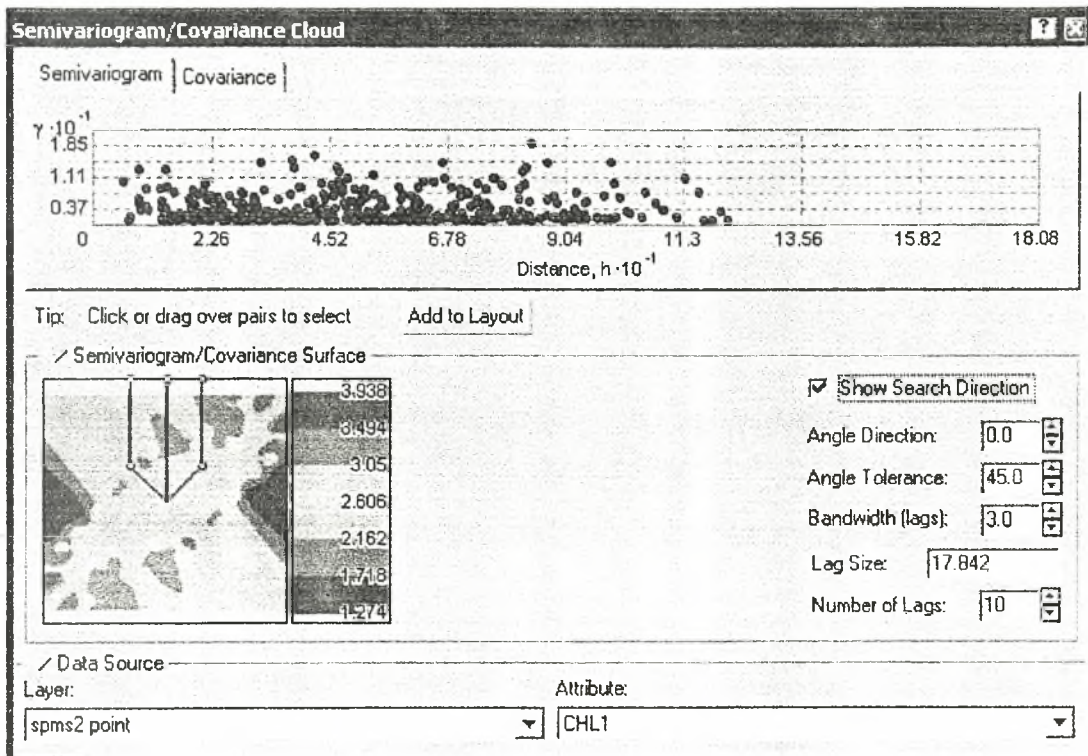
Διάγραμμα της ημιπαράλλακτικότητας των τιμών της χλωροφύλλης στα φύλλα αμπέλου (1 η Δειγματοληψία) στην περιοχή μελέτης
