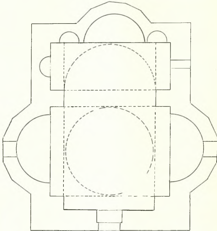
Σχέδ. 6. Σκιάθος. Καθολικὸν μονῆς Κεχρεᾶς. Κάτοπις
