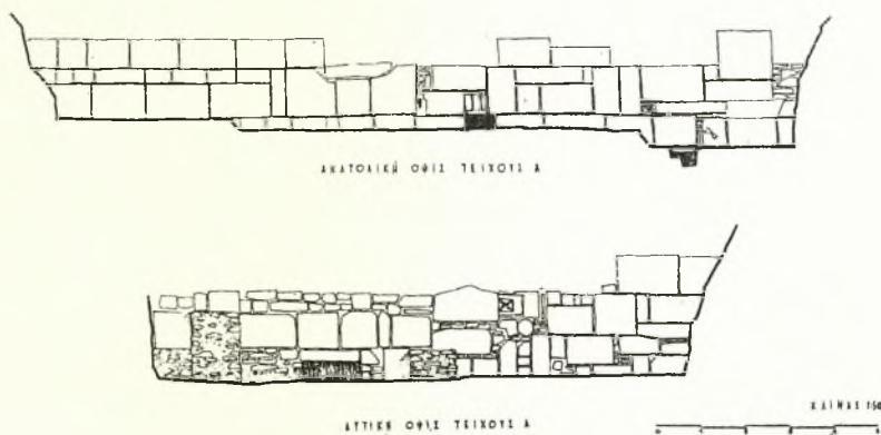
Σχέδ. 2. Χαλκίς. Αί δύο όψεις του άποκαλυφθέντος τείχους Α
