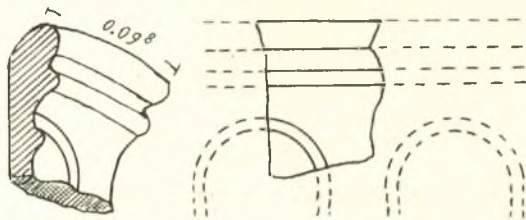
Εἰκ. 8. Τεμάχιον τραπέζης ἀγαπῶν ἢ μαρτύρων.
