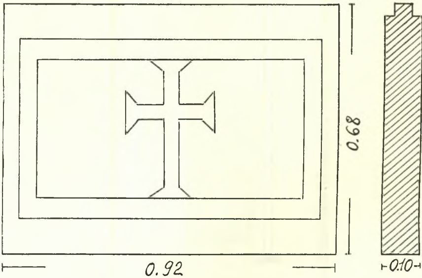
Εἰκ. 3. Πάριον θωράκιον. Ὅψις καὶ τομή.
