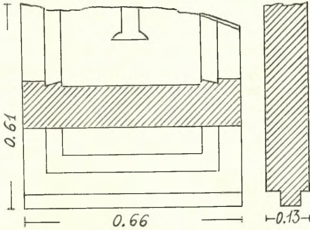
Εἰκ. 4. Πῶρινον θωράκιον. Ὅψις καὶ τομαί.
