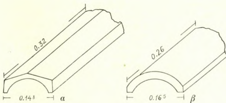
Εἰκ. 9. Πήλιναι κεραμίδες ἐκ τῆς στέγης.
