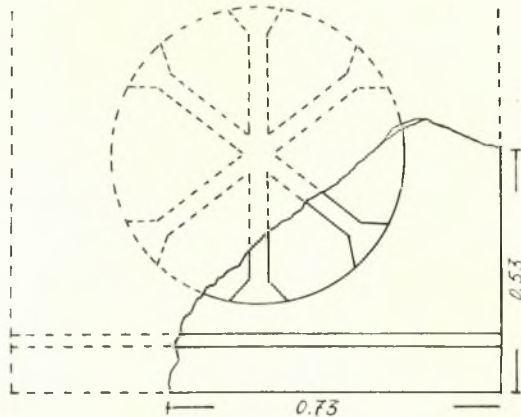
Εἰκ. 5. Θωράκιον μετὰ διακόσμησιν χρύσματος.
