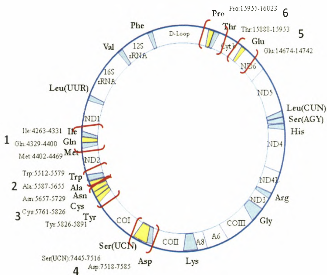
Εικόνα 15: Οι περιοχές του mtDNA που αντιστοιχούν στα ζεύγη των εκκινητών (6) που χρησιμοποιήθηκαν φαίνονται μέσα στα κόκκινα πλαίσια.
