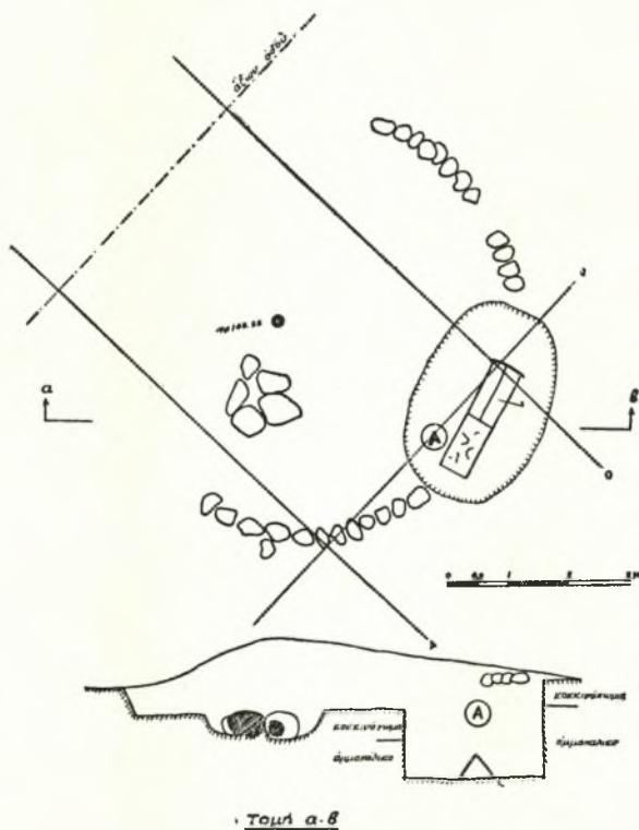
Σχεδ. 3. Ὁ τύμβος II
