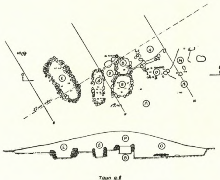
Σχεδ. 5. Τομὴ α-β τοῦ τύμβου III
