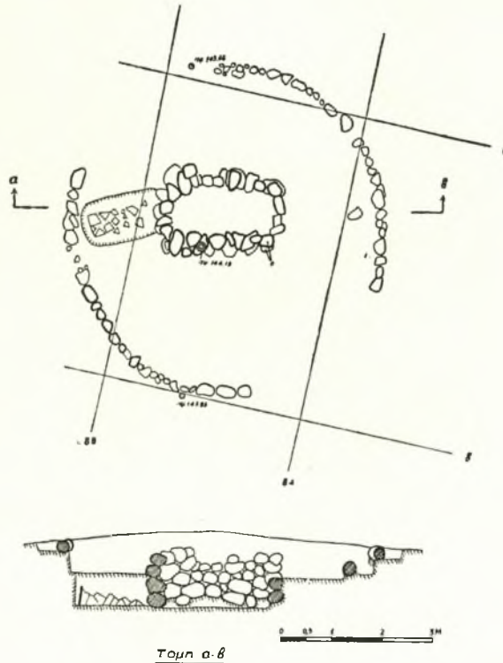
Σχ ε δ. 32. Ὁ τύμβος XXIV, κάτοψις καὶ τομὴ α-β
