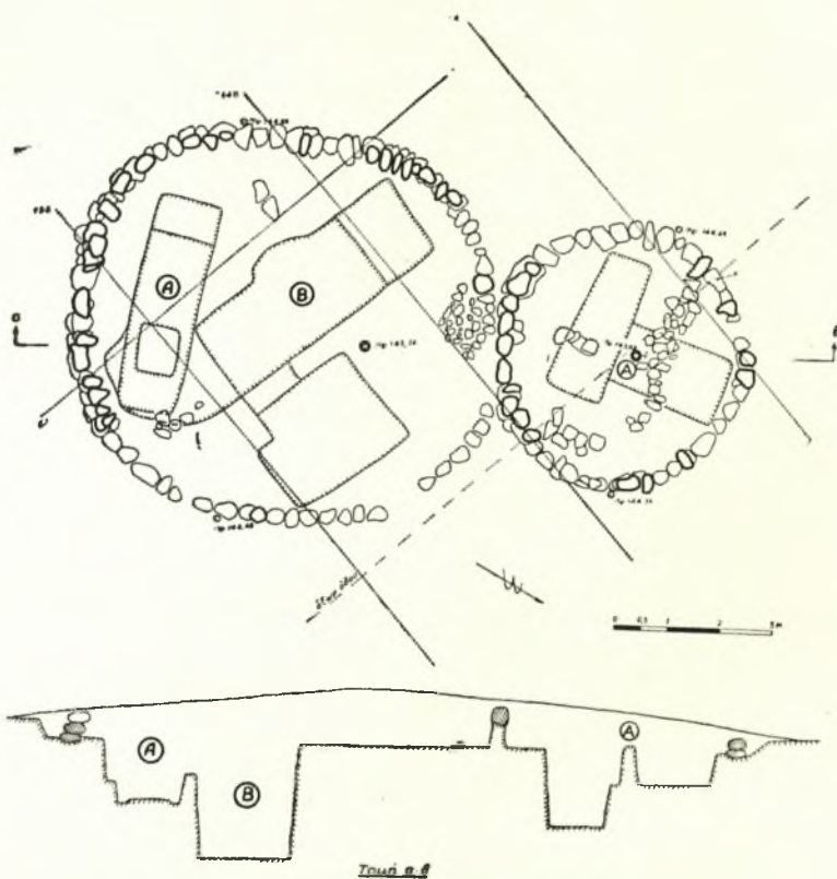
Σχεδ. 39. Ὁ τύμβος XL, κάτωτις καὶ τομὴ α-β
