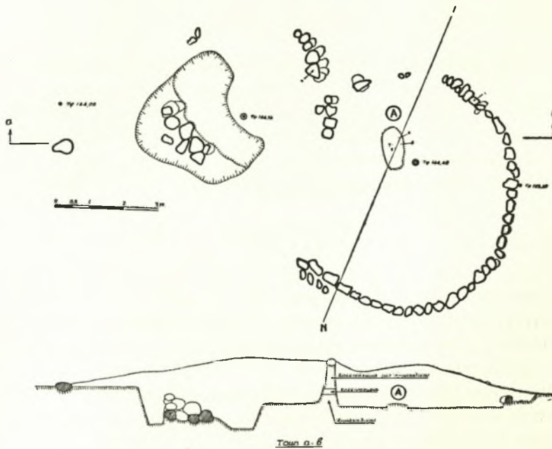
Σχεδ. 22. Ὁ τύμβος XV, κάτωφης καὶ τομὴ α-β
