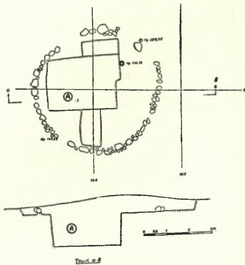
Σχεδ. 41. Ὁ τύμβος XLIV, κάτοψις και τομή α - β
