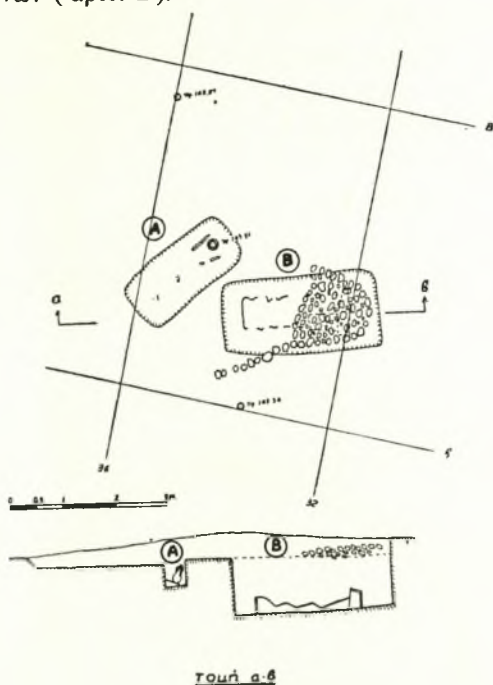
Σχεδ. 17. Ὁ τύμβος X, κάτωτις καὶ τομή α-β
