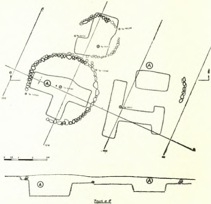
Σχεδ. 37. Ὁ τύμβος XXXVII, κάτοψις καὶ τομή α-β
