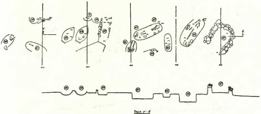
Σχεδ. 49. Τομή γ - δ τοῦ τύμβου LXV
