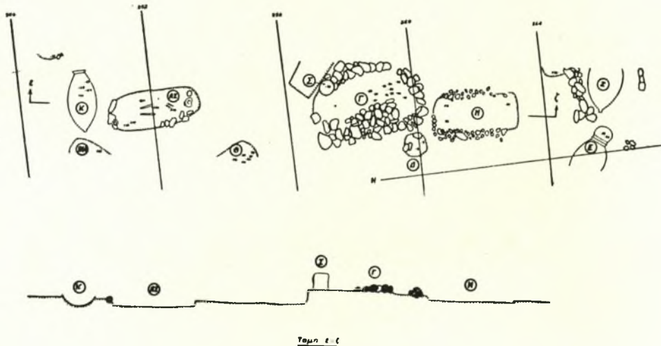
Σχεδ. 50. Τομὴ ε-ζ τοῦ τύμβου LXV
