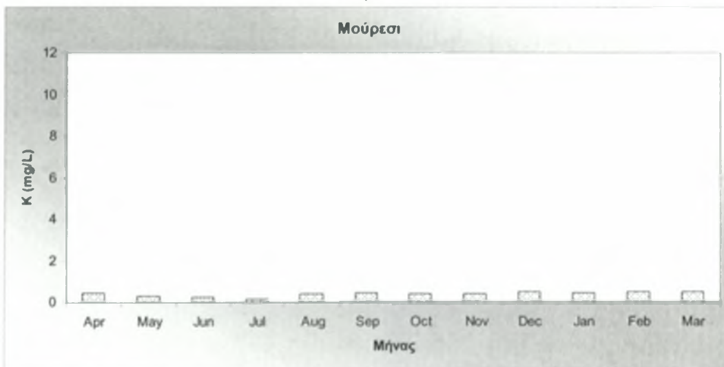
Σχήμα 3.65 Συγκέντρωσεις ιόντων α) αμμωνιακών β) νατρίου γ) καλίου κατά την περίοδο Απριλίου 2007-Μαρτίου 2008.
