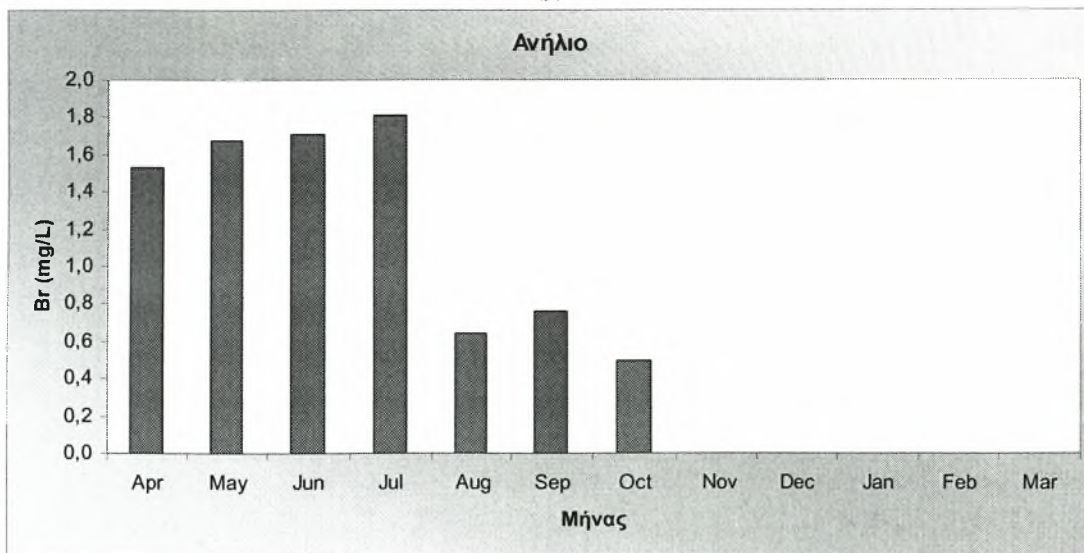
Σχήμα 3.69 Συγκέντρωσεις ιόντων α) φθορίου β) χλωρίου γ) βρωμίου κατά την περίοδο Απριλίου 2007-Μαρτίου 2008.
