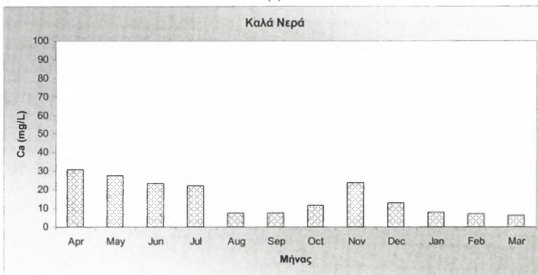
Σχήμα 3.30 Συγκέντρωσεις ιόντων α) μαγνησίου β) ασβεστίου κατά την περίοδο Απριλίου 2007-Μαρτίου 2008.
