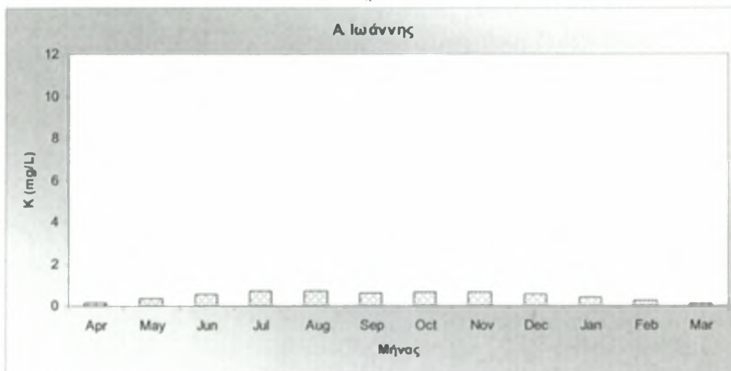
Σχήμα 3.41 Συγκέντρωσεις ιόντων α) αμμωνιακών β) νατρίου γ) καλίου κατά την περίοδο Απριλίου 2007-Μαρτίου 2008.
