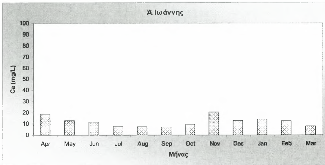
Σχήμα 3.42 Συγκέντρωσεις ιόντων α) μαγνησίου β) ασβεστίου κατά την περίοδο Απριλίου 2007-Μαρτίου 2008.
