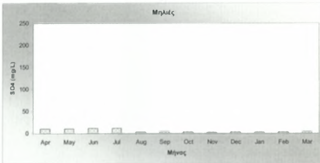
Σχήμα 3.52 Συγκέντρωσεις ιόντων α) νιτρωδίων β) νιτρικών γ) θειικών κατά την περίοδο Απριλίου 2007-Μαρτίου 2008.
