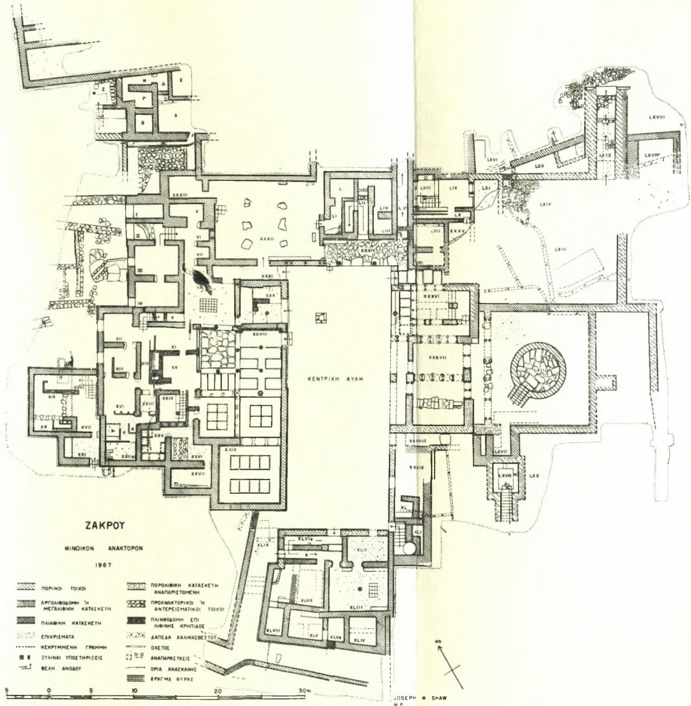
Γενικόν σχέδιον κατόψεως τοῦ ἀνακτόρου Ζάχρου.
