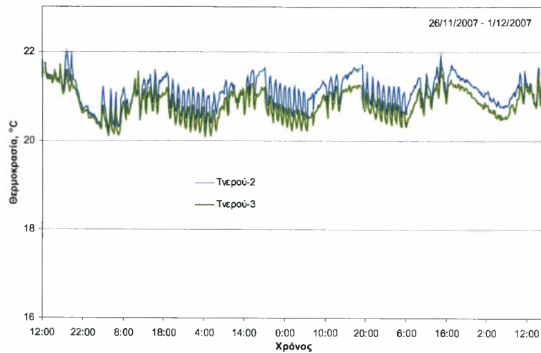
Σχήμα 4.1.2. Πορεία των τιμών της θερμοκρασίας του νερού στο εσωτερικό των σωλήνων από 26/11 έως 01/12/2007.
