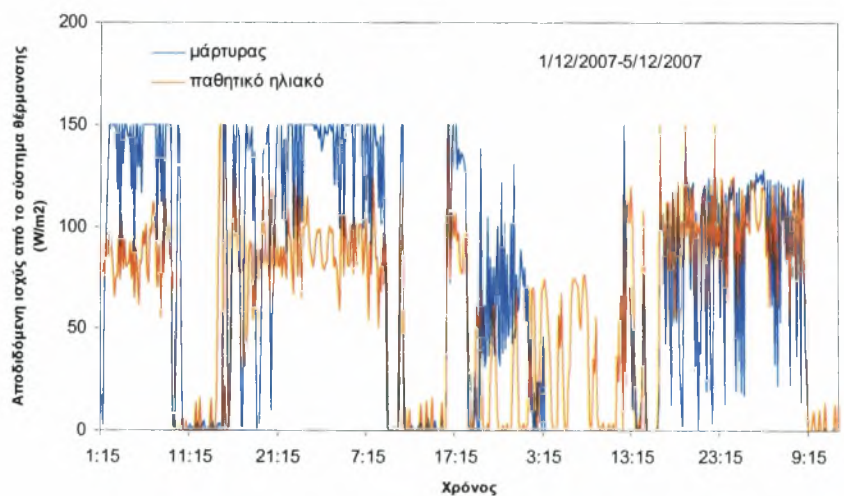
Σχήμα 4.1.5. Πορεία των τιμών της αποδιδόμενης ισχύος από το σύστημα θέρμανσης για τη θέρμανση των δύο θερμοκηπίων κατά τη διάρκεια της χειμερινής περιόδου των μετρήσεων.
