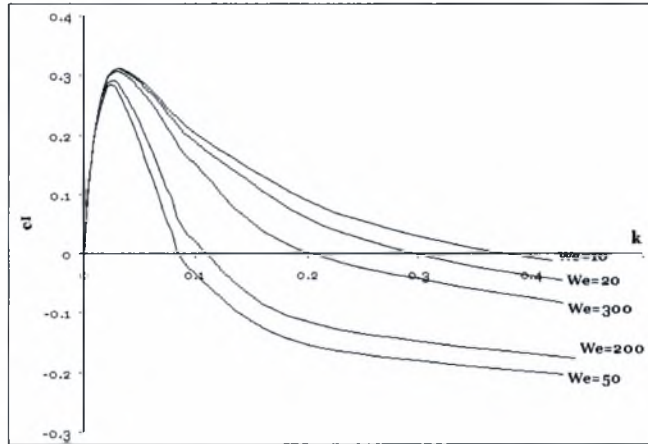
Σχήμα 4.3. Μεταβολή του φανταστικού μέρους της φασικής ταχύτητας για \varphi=5^\circ , Re=30 .
