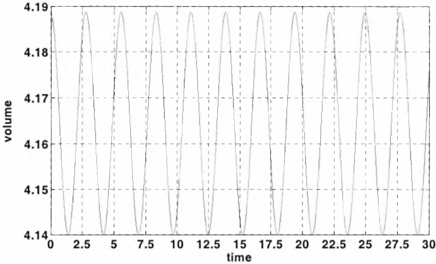
Σχήμα 2. Ο όγκος της μικροφουσαλίδας σα συνάρτηση του χρόνου για γραμμική διαταραχή. Δεδομένα προσομοίωσης: R_{bal}=1.5 \mu\text{m} , G_s=18 \text{ MPa} , \alpha=0.5 , \delta=15 \text{ nm} , \rho_l=998 \text{ kg/m}^3 , P_{st}=1 \text{ atm} , \nu_f=2.4 \text{ MHz} , \varepsilon_{inf}=0.05 , \gamma=1.4 , αριθμός στοιχείων 60.
