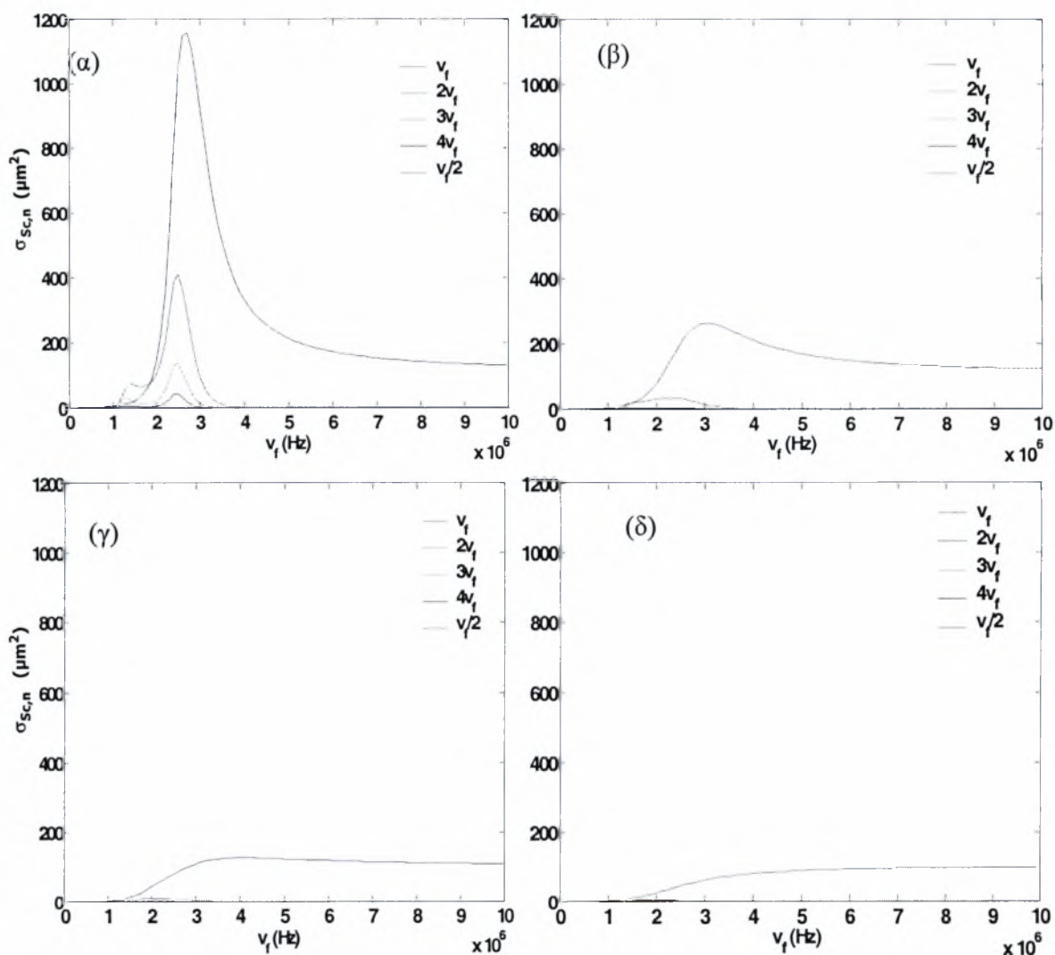
Σχήμα 6. Το \sigma_{Sc,n} σε συνάρτηση της εξωτερικής συχνότητας για α) \mu_s=0.6 \text{ kgm}^{-1}\text{s}^{-1} β) \mu_s=1.6 \text{ kgm}^{-1}\text{s}^{-1} , γ) \mu_s=2.6 \text{ kgm}^{-1}\text{s}^{-1} , δ) \mu_s=3.6 \text{ kgm}^{-1}\text{s}^{-1} . Δεδομένα προσομοίωσης: \gamma=1.4 , P_{inf}=101325 \text{ Pa} , \rho_l=998 \text{ kg/m}^3 , s_1=0.04 \text{ kg/s}^2 , s_2=0.005 \text{ kg/s}^2 , \mu_l=0.001 \text{ kgm}^{-1}\text{s}^{-1} , C_l=1500 \text{ m/s} , G_s=35 \text{ MPa} , \alpha=3 \cdot 10^{-6} \text{ m} , \delta=15 \cdot 10^{-9} \text{ m} , E_{inf}=2.05 . u_r(t=0)|_{r=1} = u_r(t=0)|_{r=a_{bul}} = 0
