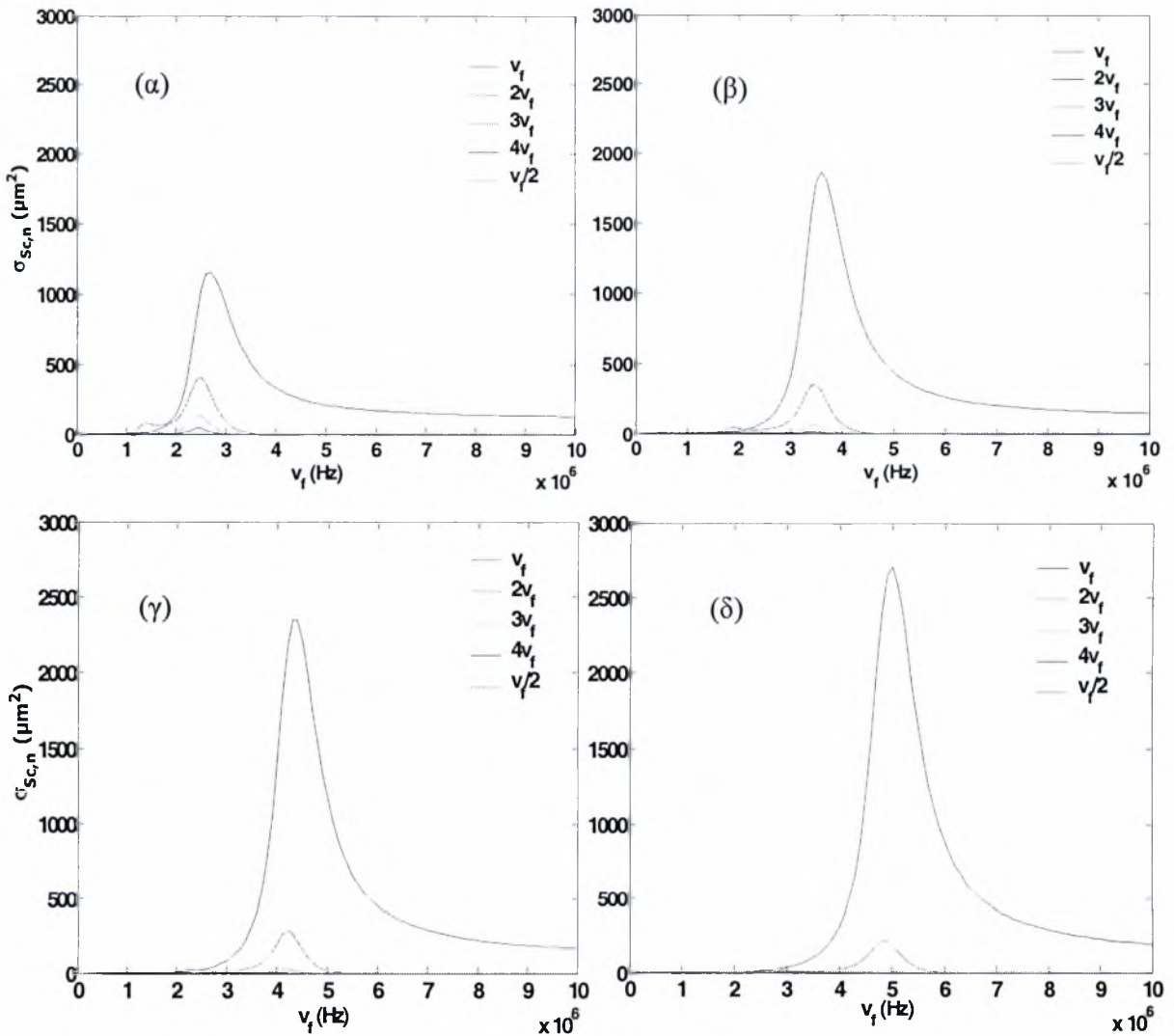
Σχήμα 5. Το \sigma_{Sc,n} σε συνάρτηση της εξωτερικής συχνότητας για α) G_s=35 MPa, β) G_s=70 MPa, γ) G_s=105 MPa, δ) G_s=140 MPa. Δεδομένα προσομοίωσης: \gamma=1.4 , P_{inf}=101325 Pa, \rho_l=998 kg/m 3 , s_1=0.04 kg/s 2 , s_2=0.005 kg/s 2 , \mu_l=0.001 kgm -1 s -1 , C_l=1500 m/s, \mu_s=0.6 kgm -1 s -1 , \alpha=3 \cdot 10^{-6} m, \delta=15 \cdot 10^{-9} m, E_{inf}=2.05 . u_r(t=0)|_{r=1} = u_r(t=0)|_{r=a_{bal}} = 0
