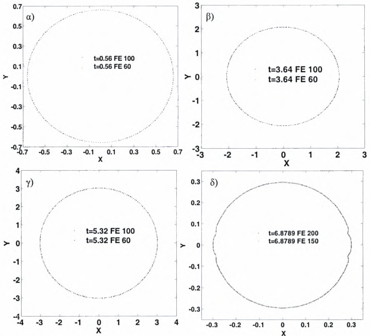
Σχήμα 4. Η ανεξαρτησία της λύσης με την πυκνωση του πλέγματος. Δεδομένα προσομοίωσης: R_{bal}=1.5 \mu m , G_s=18 MPa , \alpha=0.5 , \delta=15 nm , \rho_l=998 kg/m^3 , P_{st}=1 atm , \nu_l=2.4 MHz , \epsilon_{inf}=12 , \gamma=1.4 .
