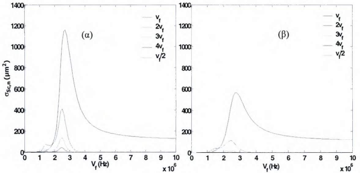
Σχήμα 8. Το \sigma_{sc,n} σα συνάρτηση της εξωτερικής συχνότητας για α) νερό ( C_I=1500 m/s, \mu_I=0.001 kgm -1 s -1 ) β) αίμα ( C_I=500 m/s, \mu_I=0.004 kgm -1 s -1 ). Δεδομένα προσομοίωσης: \gamma=1.4 , P_{inf}=101325 Pa, \rho_I=998 kg/m 3 , s_1=0.04 kg/s 2 , s_2=0.005 kg/s 2 , \alpha=3 \cdot 10^{-6} m, G_s=35 MPa, \mu_s=0.6 kgm -1 s -1 , \delta=15 \cdot 10^{-9} m, E_{inf}=2.05 . u_r(t=0)|_{r=1} = u_r(t=0)|_{r=a_{bul}} = 0
