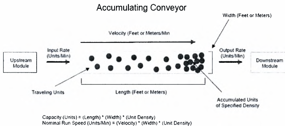
Σχήμα 3-4: Ιμάντας Συγκέντρωσης
