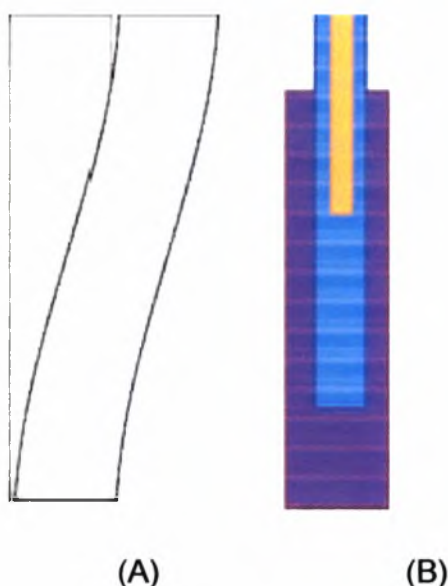
Σχήμα 2.17 Σχηματική απεικόνιση των δύο πιθανών τρόπων παραμόρφωσης και αστοχίας των νανοσωληνών. (A) Λυγισμός σε μια λεπτή στήλη. (B) Τηλεσκοπική ενός Πολύτοιχου νανοσωληνά. Η θραύση των νανοσωληνών είναι ο τρίτος τρόπος, αλλά δεν εμφανίζεται στο σχήμα.
