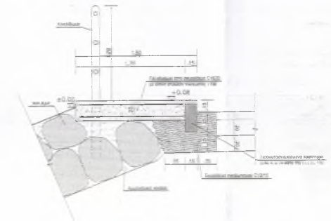
Απτόμωρο 5Γ ΚΑ. 1:20
