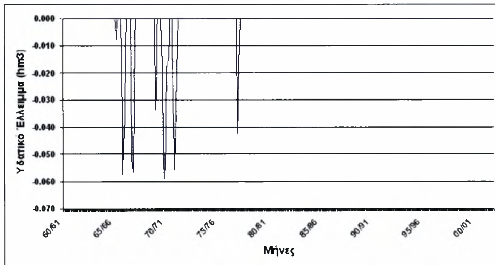
Σχήμα 6.2.8 Μηνιαίο υδατικό ισοζύγιο του ταμιευτήρα Μαυρομάτη
