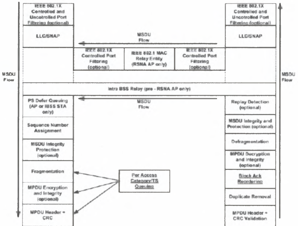
Εικόνα 2.2. Αρχιτεκτονική MAC.
