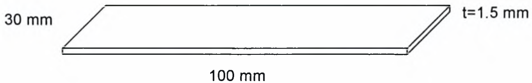
Εικόνα 3.2 – Δοκίμιο Συγκόλλησης
