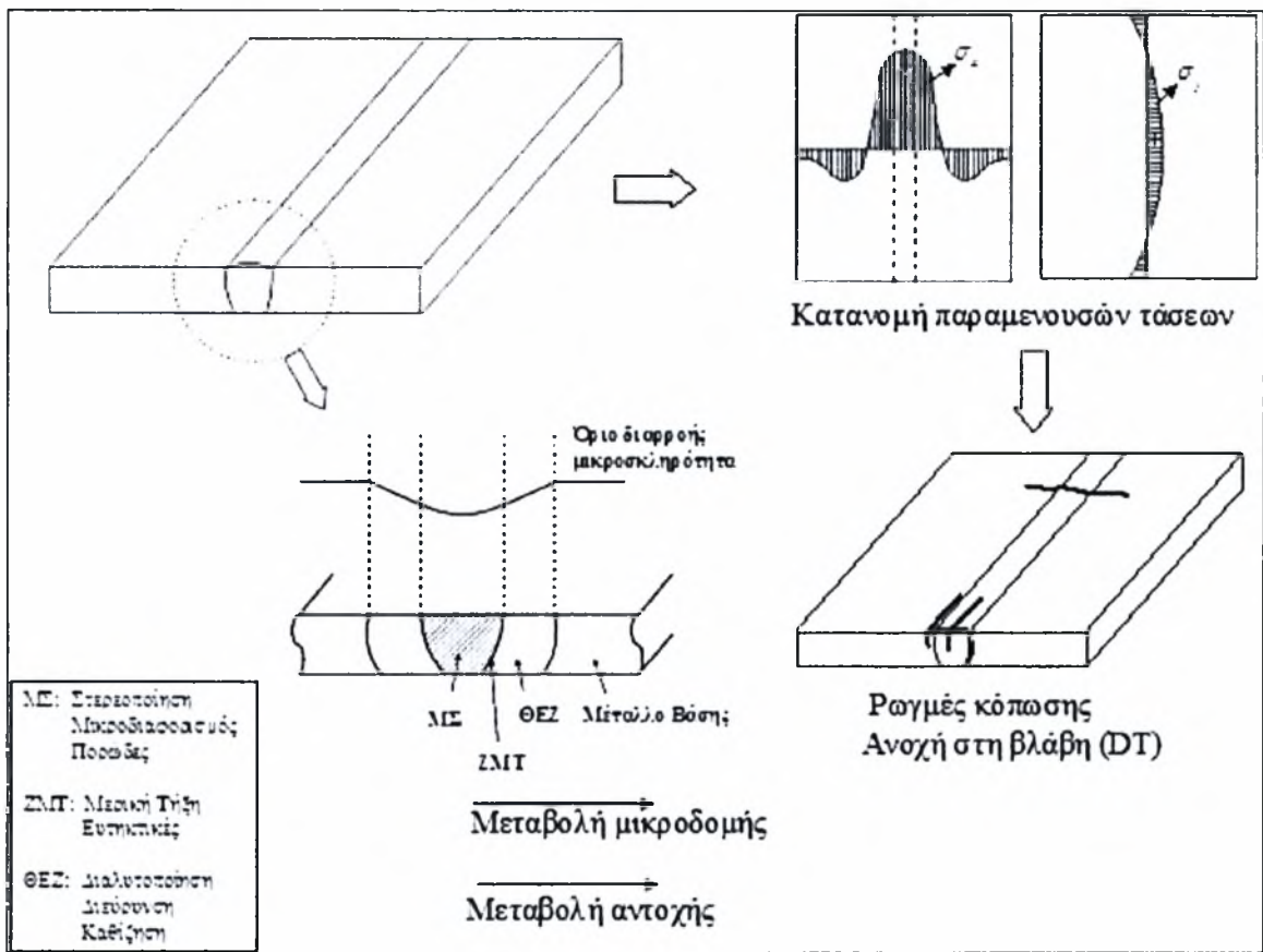
Εικόνα 1.3 – Απλοποιημένη σχηματική παράσταση συγκόλλησης συμβολής σε κράμα Al : Η επίδραση της μεταβολής της μικροδομής στη συγκόλληση (ΜΣ, ZMT, ΘΕΖ) καθώς και των παραμενουσών τάσεων.
