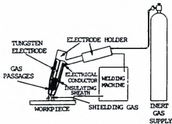
Εικόνα 2-1 – Τυπικό Setup για Συγκόλληση με την Μέθοδο TIG
